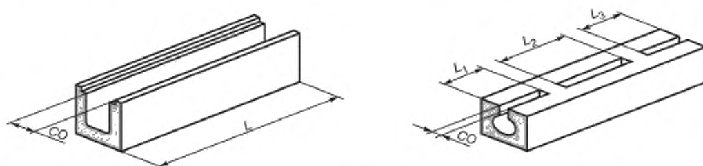
Площадь просвета = CO \cdot L , L = L_1 + L_2 + L_3
