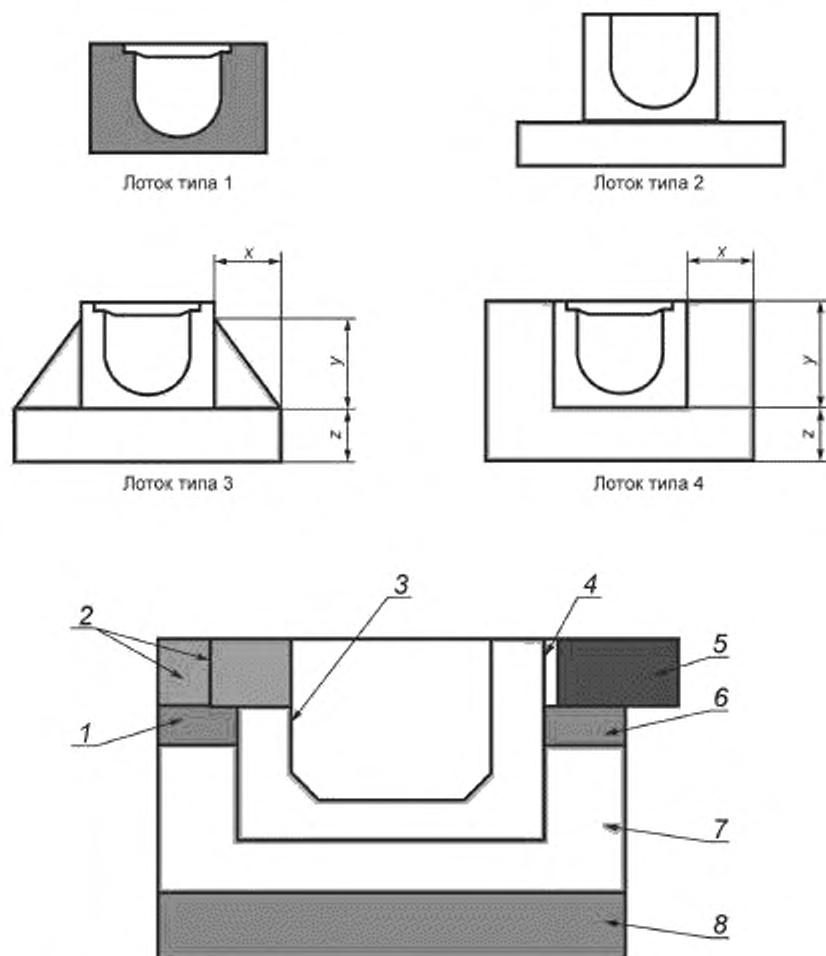
х, у и z — геометрические размеры несущего фундамента и обмуровки 1 — подстилающий слой; 2 — штучные элементы мощения; 3 — лоток; 4 — битумная мастика; 5 — дорожное покрытие; 6 — верхний слой основания; 7 — основание из бетона; 8 — подстилающий слой
