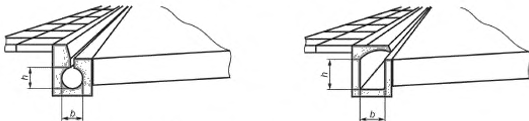
h , b — внутренние размеры (смачиваемый периметр)
