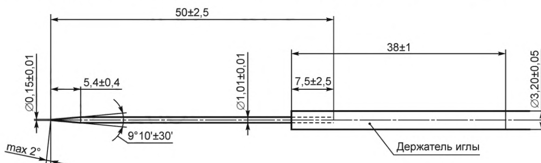
Рисунок 1 — Пенетрационная игла
