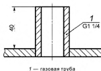
Рисунок Б.3 — Штуцер для измерения давления газа
