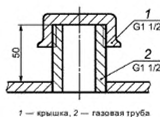
Рисунок Б.2 — Штуцер для измерения температуры газа
