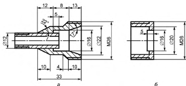
Рисунок Г.2 — Патронодержатель
