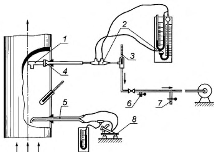
1 — патрон со стекловолокном; 2 — реометр; 3 — термометр; 4 — патрондержатель; 5 — напорная трубка; 6 — подсос воздуха; 7 — сбор конденсата; 8 — микроанометр
