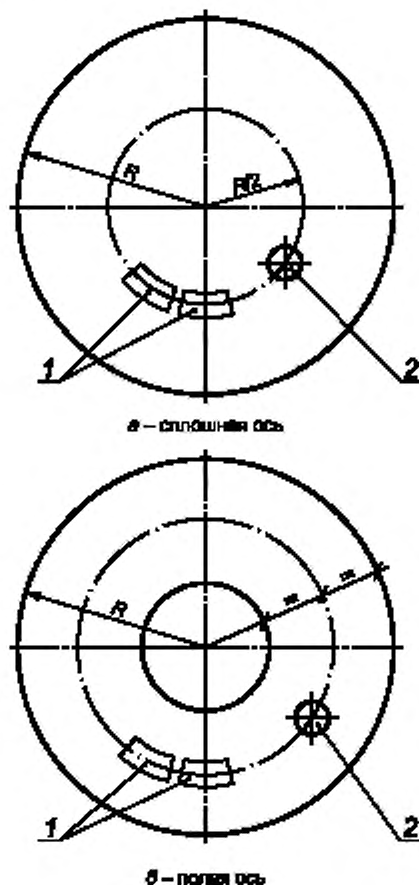
Рисунок 4 — Положение заготовок образцов для испытаний стали осей на механические свойства
