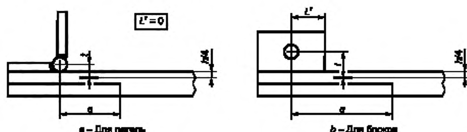
Рисунок 4 — Схема ввода нагрузки раскрытия по отношению к образцу ДКБ L' — половина ширины блока нагрузки, a — длина трещины (в процессе испытания); h — толщина образца; t — параметр расстояния
