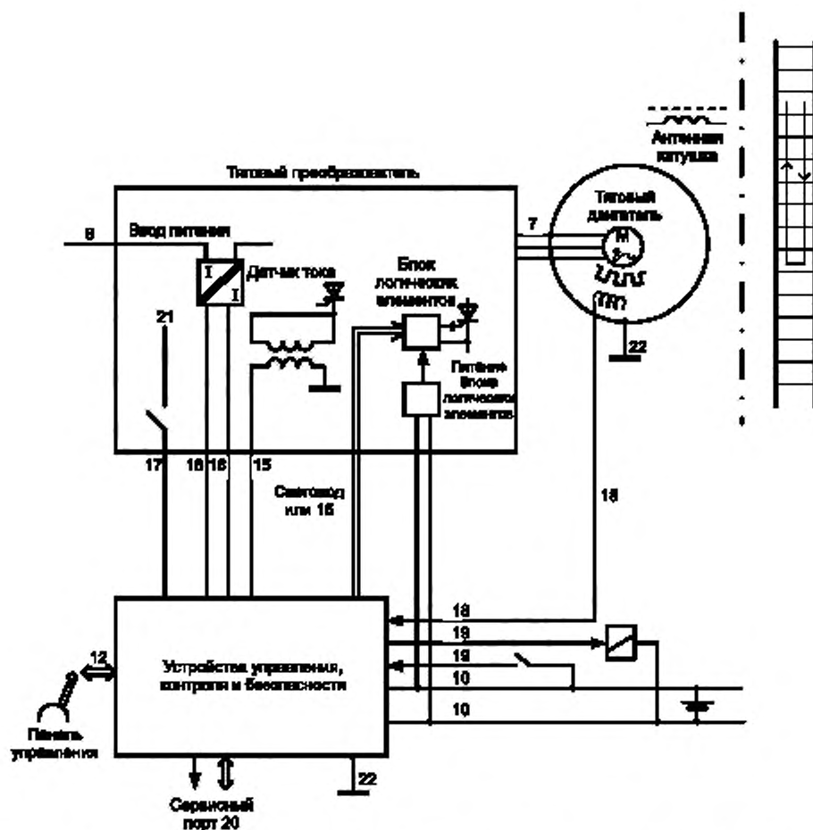
Рисунки А.8 — Дополнительные порты тягового преобразователя тока и электронных схем управления
