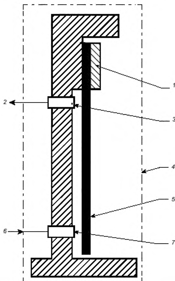
1 — зажим; 2 — к усилителю; 3 — детектор; 4 — камера с регулируемой температурой; 5 — образец; 6 — от генератора колебаний; 7 — устройство возбуждения
