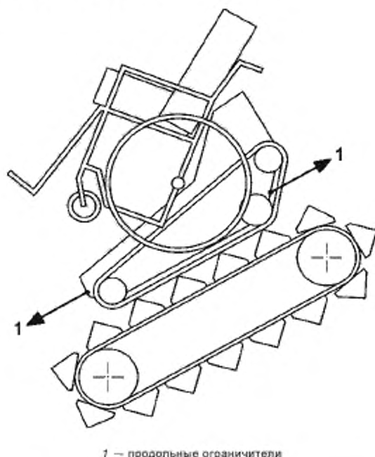
Рисунок F.1 — Самоустанавливающееся устройство для преодоления лестниц на эскалаторной испытательной машине
