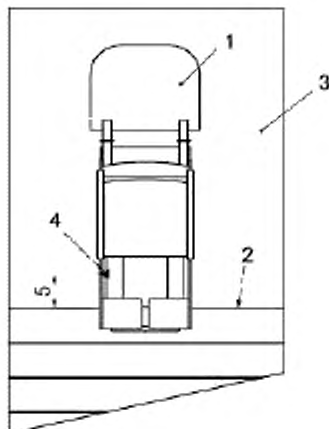
1 — ограничитель пространства для сопровождающего; 2 — оковка ступени под номером 8; 3 — верхняя лестничная площадка; 4 — базовая метка; 5 — расстояние между оковкой ступени под номером 8 и базовой меткой
