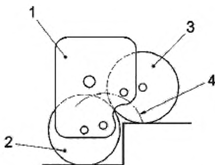
Рисунок 10 — Пример двухтактного механизма преодоления
