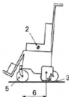
е) Двухтактный механизм преодоления
