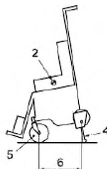
f) Трехтактный механизм преодоления
