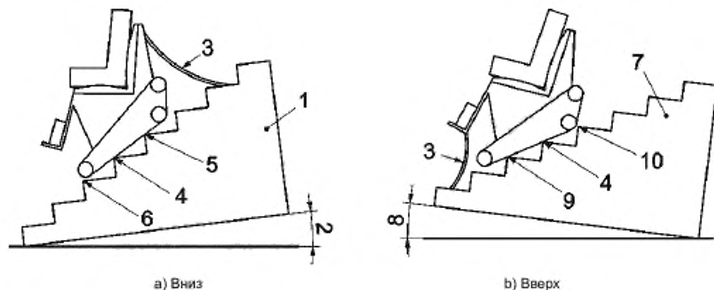
1 — испытательная лестница, наклоненная вперед; 2 — угол наклона вперед испытательной лестницы; 3 — провисающая веревка, ограничивающая перевертывание; 4 — ступень под номером 4, действующая как ось наклона; 5 — ступень выше ступени под номером 4, на которой обнаружена потеря контакта; 6 — ступень ниже ступени под номером 4, на которой обнаружен контакт; 7 — испытательная лестница, наклоненная назад; 8 — угол наклона назад испытательной лестницы; 9 — ступень ниже ступени под номером 4, на которой обнаружена потеря контакта; 10 — ступень выше ступени под номером 4, на которой обнаружен контакт
