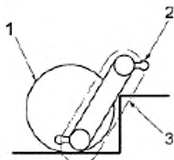
1 — нижний исполнительный механизм (колесо); 2 — верхний исполнительный механизм (палец); 3 — траектория самой нижней точки пальца относительно механизма преодоления
