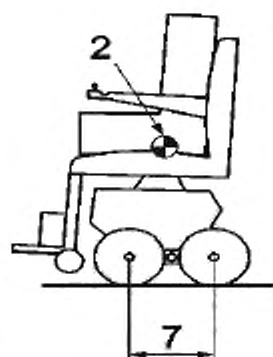
g) Динамически контролируемое устройство для преодоления лестниц
