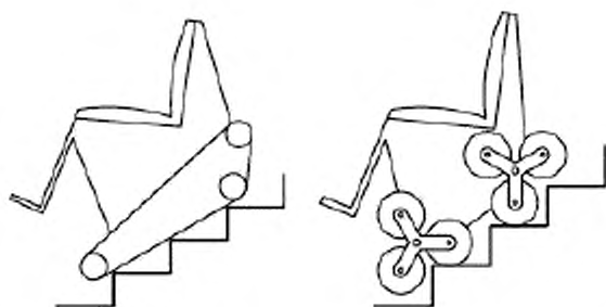
Рисунок А.5 — Представители типичных самоустанавливающихся устройств для преодоления лестниц с креслом, управляемых пользователями (тип Е)
