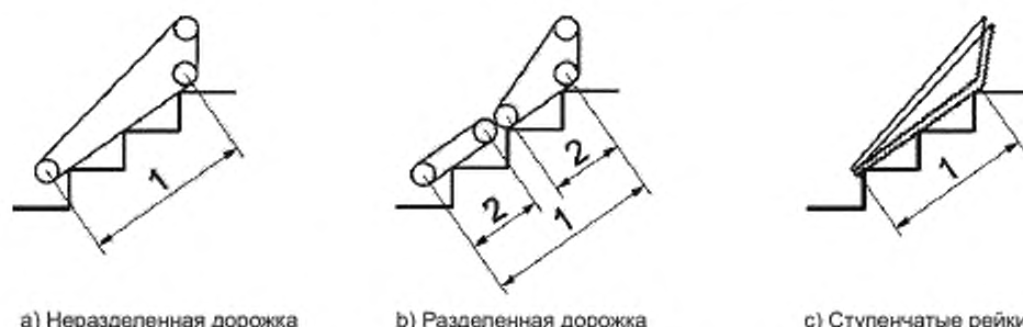
1 — общая длина площади контакта со ступенями непрерывного механизма преодоления; 2 — длина секции площади контакта со ступенями одной секции разделенного непрерывного механизма преодоления
