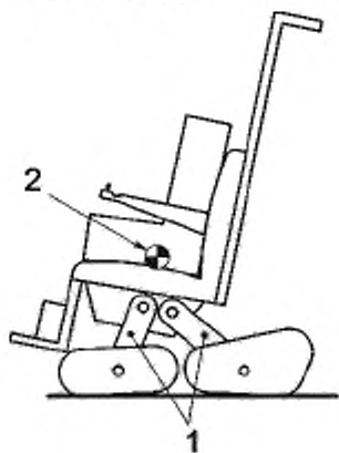
а) Гусеницы на кронштейнах
