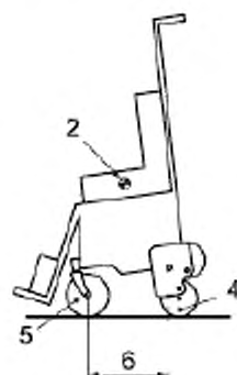
е) Двухтактный механизм преодоления
