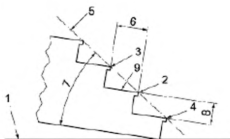
1 — горизонтальная испытательная плоскость; 2 — оковка измеряемой ступени, 3 — оковка следующей более высокой ступени; 4 — оковка следующей более низкой ступени; 5 — линия наклона; 6 — ширина ступени (3.20); 7 — угол наклона (3.34); 8 — высота ступени (3.37); 9 — проступь (3.51)
