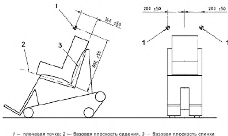
Рисунок 7 — Размещение плечевых точек
