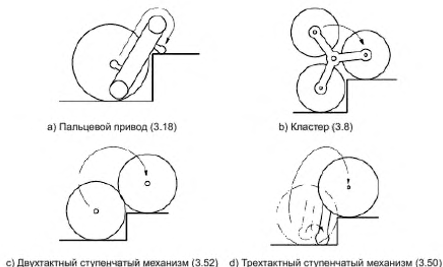
Рисунок 8 — Примеры ступенчатых механизмов преодоления
