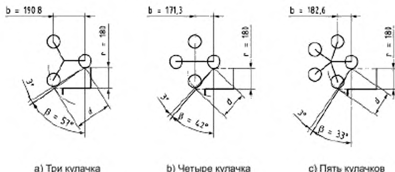
Рисунок К.2 — Длины d и b (примеры для n = 3, 4 и 5 )
