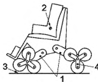
б) Кластеры на кронштейнах
