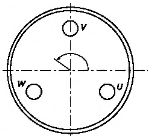
Рисунок Л.1 — Схема расположения нижних выводных концов верхних и средней секций
