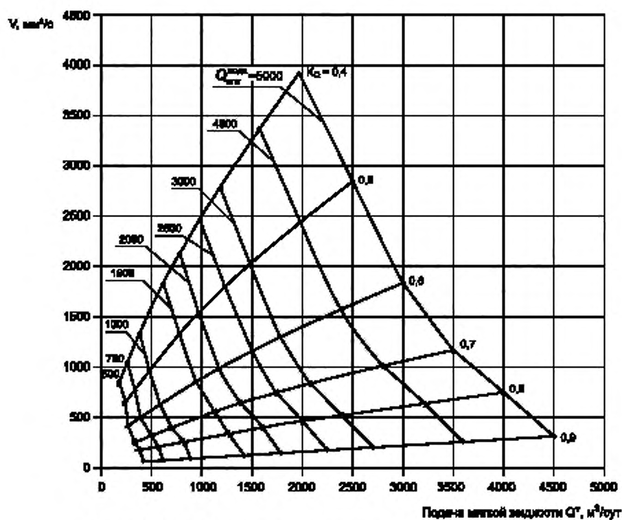
Рисунок А.1 — График изменения оптимальной подачи центробежного и диагонального насоса ( Q_{\text{опт}}^0 = 500 - 5000 \text{ м}^3/\text{сут} )
