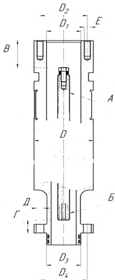
Рисунок К.1 — Габаритные и присоединительные размеры гидрозакит с диаметром корпуса 69; 81; 86; 92; 103; 114 мм
