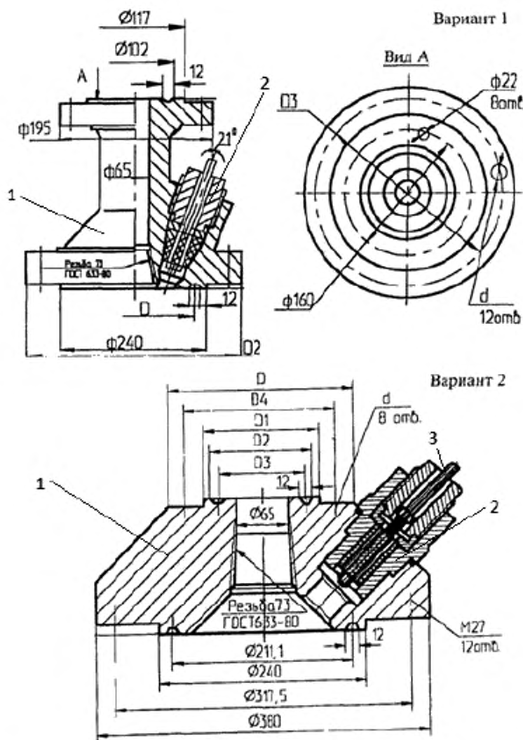
1 — переходник трубной головки; 2 — электрический пенетратор; 3 — жилы кабельной линии. Размеры представлены для примера
