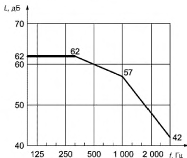
Рисунок 1 — Оценочная кривая для ударного шума (третьоктавные полосы)
