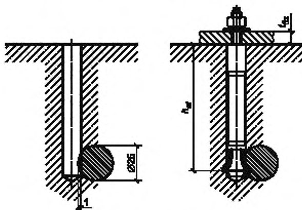
Рисунок 2 — Схема испытания анкера при влиянии армирования основания
