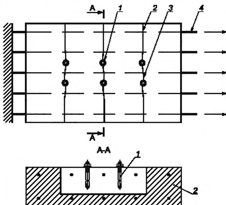
1 — анкер; 2 — инициатор трещины; 3 — трещина; 4 — арматура
