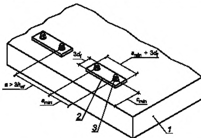
Рисунок А.4 — Испытание на проверку минимальных межосевых и краевых расстояний
