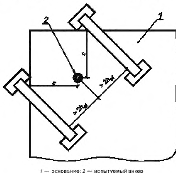
Рисунок 1 — Пример оснастки для испытаний на растяжение анкеров, установленных в углу
