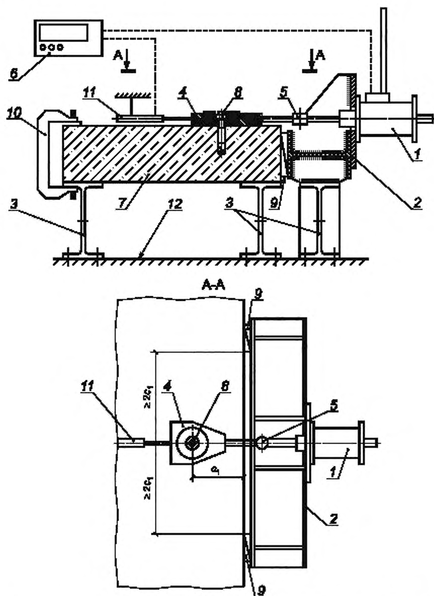
1 — домкрат с датчиком усилия (давления); 2 — силовая рама; 3 — опора, закрепленная к силовому полу; 4 — универсальное захватывающее устройство с тягой; 5 — шарнир; 6 — устройство регистрации контрольных параметров (силы, перемещения); 7 — основание; 8 — испытуемый анкер; 9 — упоры; 10 — трубушина; 11 — индикатор перемещения на независимом штативе; 12 — силовой пол
