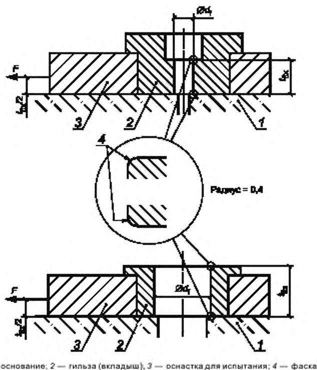
Рисунок А.3 — Гильза для испытания на сдвиг
