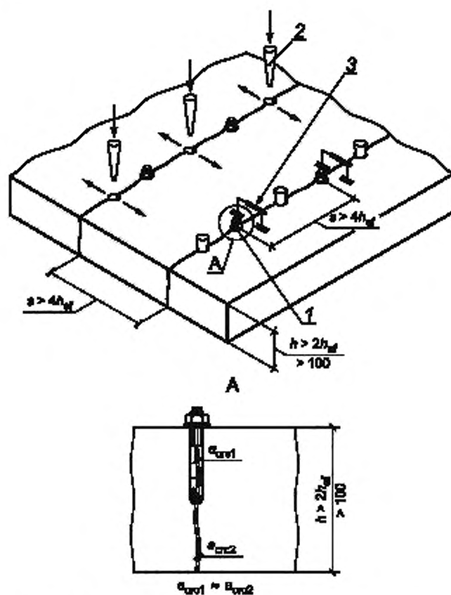
Рисунок А.5 — Испытание в основании с трещиной
