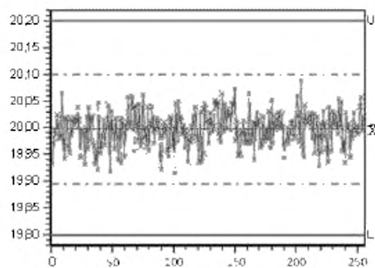
б) Пример временной диаграммы модели A1
