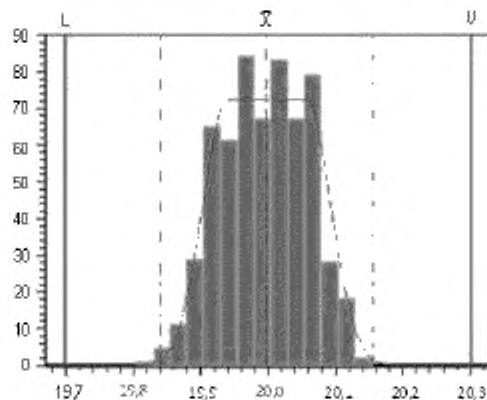
в) Пример гистограммы модели С3
