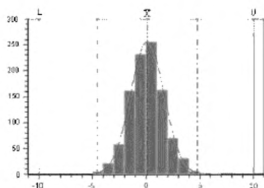
с) Пример гистограммы модели С1
