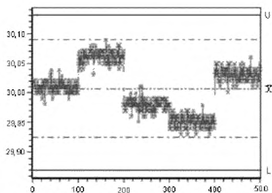
б) Пример временной диаграммы модели С4
