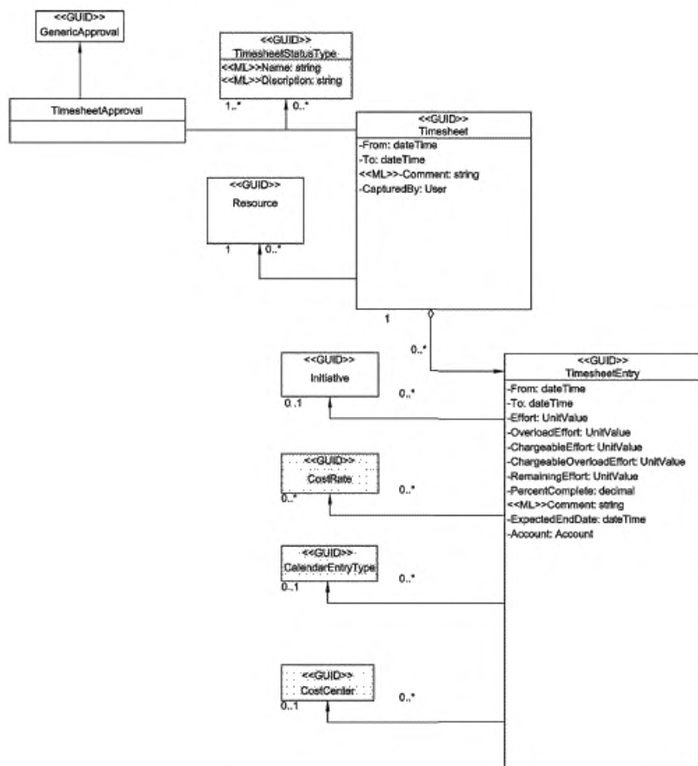
Рисунок 8 — Управление ресурсами
