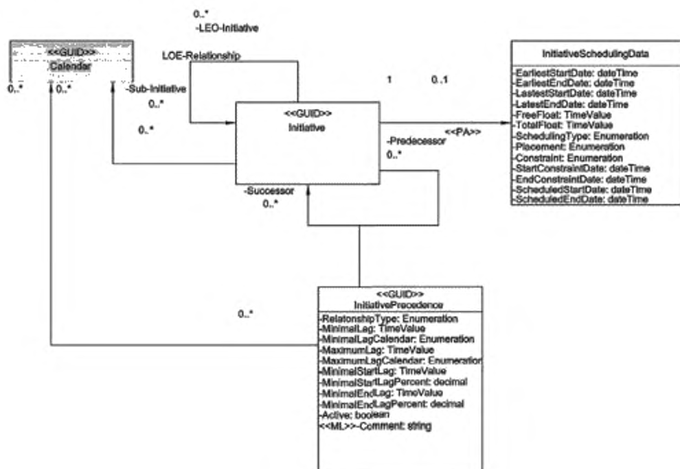
Рисунок 5 — Управление сроками
