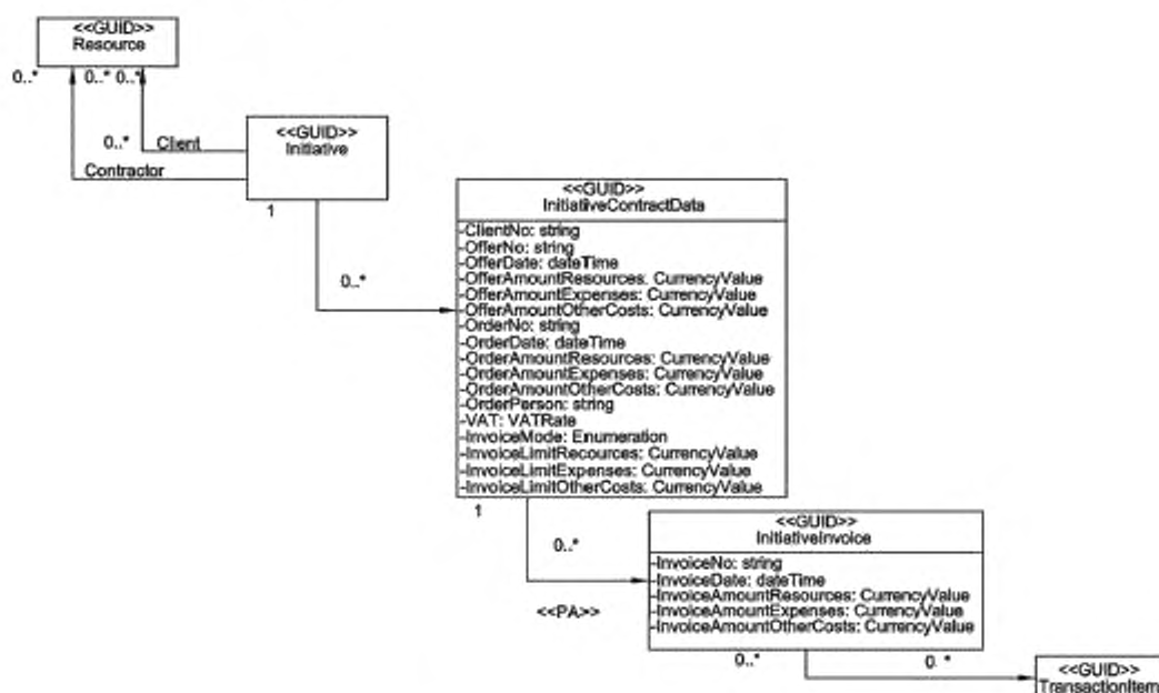
Рисунок 4 — Управление закупками
