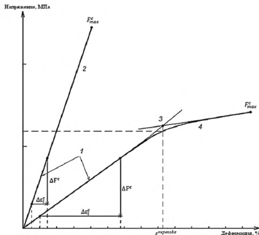
1 — диапазон определения модуля упругости и коэффициента Пуассона; 2 — линейная диаграмма деформирования; 3 — точка перехода; 4 — диаграмма деформирования с двумя линейными участками
