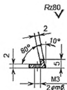
Рисунок А.7 — Ролик (см. рисунок А.1, 6)
