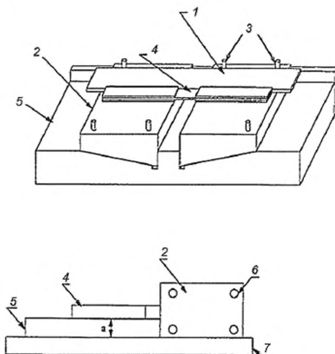
1 — прокладка; 2 — клиновые захваты; 3 — штифты; 4 — образец; 5 — основание; 6 — зажимные винты; 7 — установочная плита Рисунок Б.3 — Примеры выравнивания образца в приспособлении с клиновыми захватами
