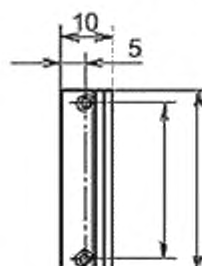
Рисунок А.9 — Стяжка (см. рисунок А.1, 8)
