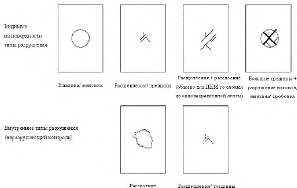
Рисунок 9 — Типовые повреждения в результате удара
