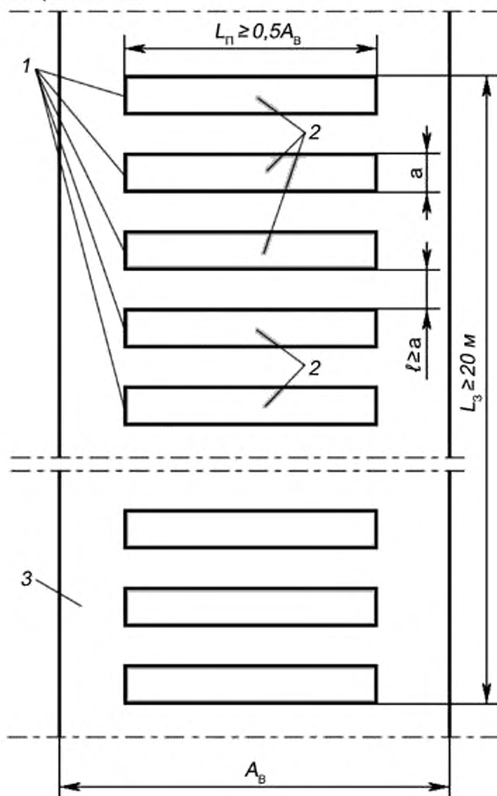
1 — полки сланцевого заслона; 2 — инертная пыль; 3 — горная выработка; L_з — длина сланцевого заслона; L_п — длина полки сланцевого заслона; \ell — расстояние между полками сланцевого заслона; A_в — ширина выработки
