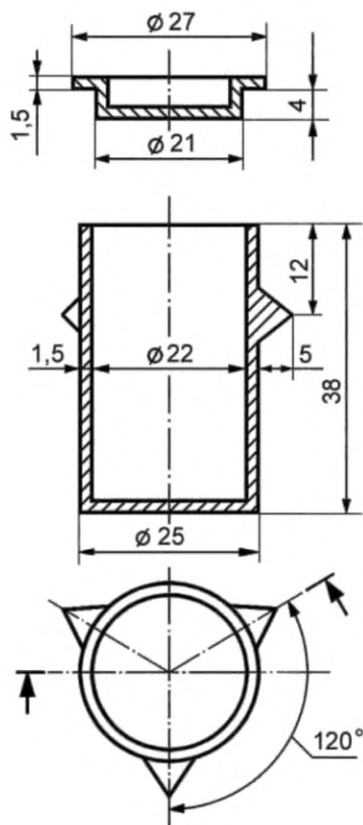
Рисунок 2 — Кварцевый тигель с крышкой
