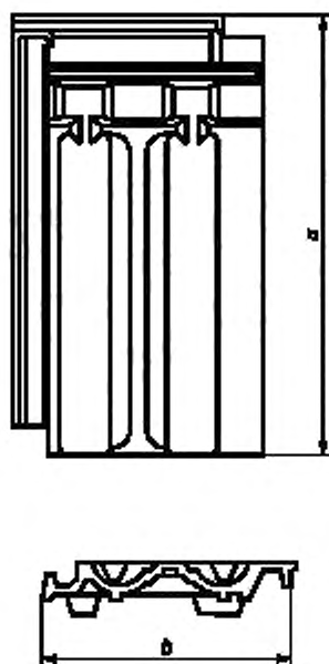
Рисунок А.1 — Пазовая (двухфальцевая) черепица
