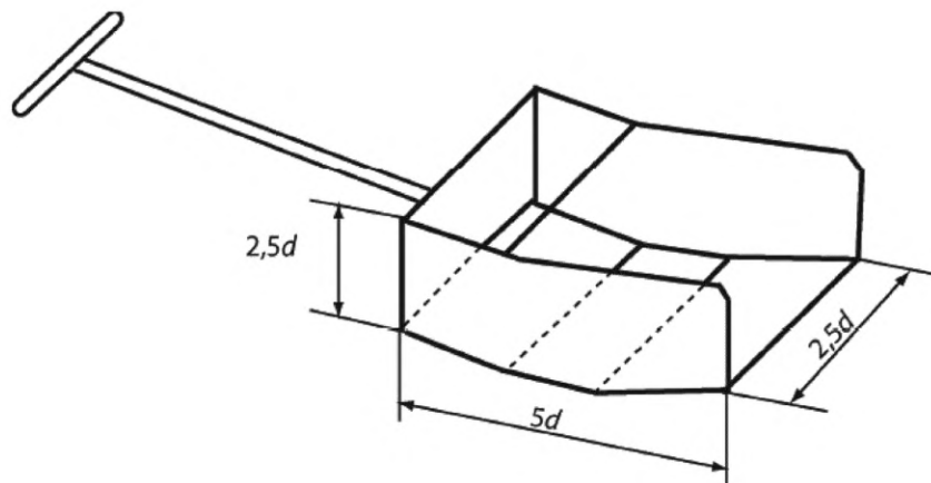
Рисунок 4 — Образец лопаты
