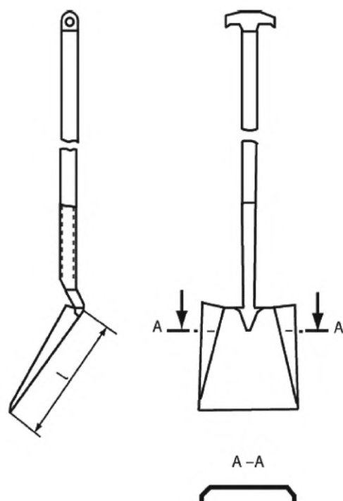
Рисунок 5 — Образец совка
