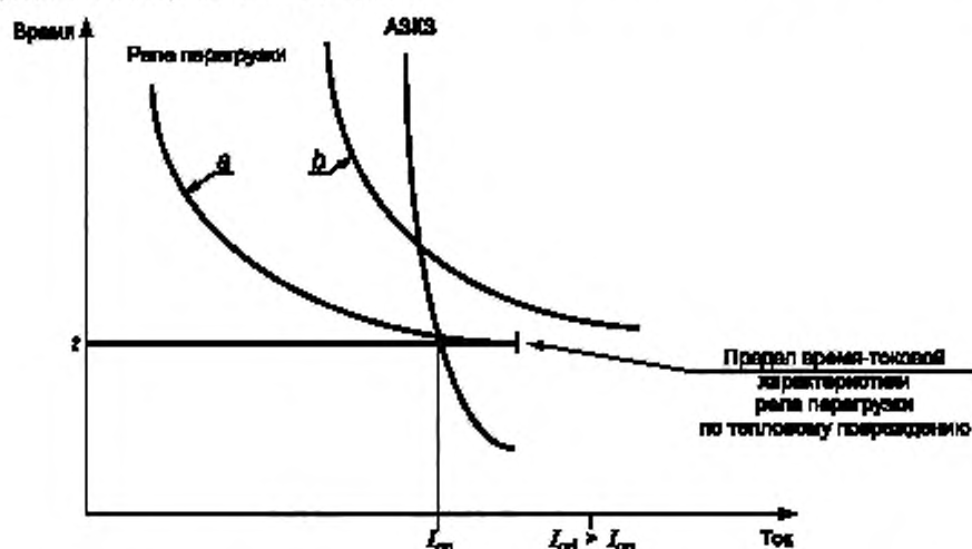
а) Координация с предохранителем
