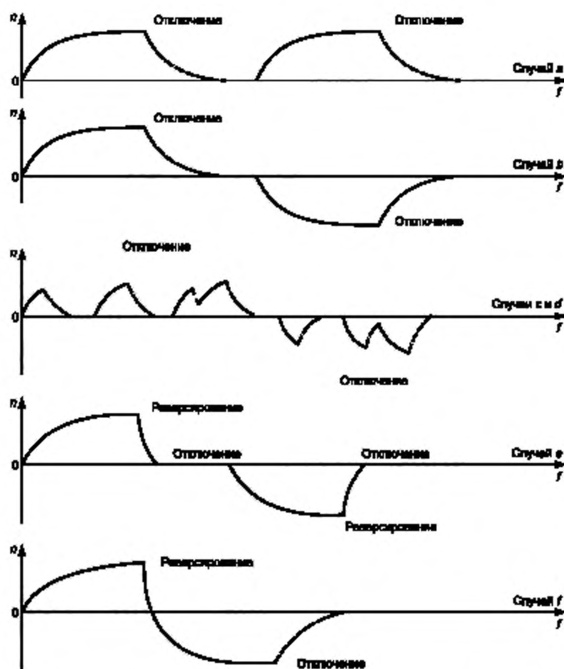
Рисунок 6 — Примеры кривых скорость — время, соответствующие случаям а)–ф) по 4.3.5.5 (пунктирные участки кривых обозначают периоды обесточивания двигателя)
