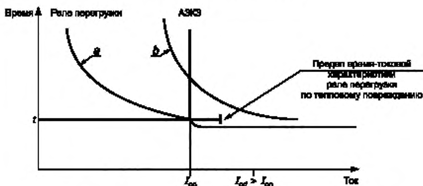
а) Координация с предохранителем
