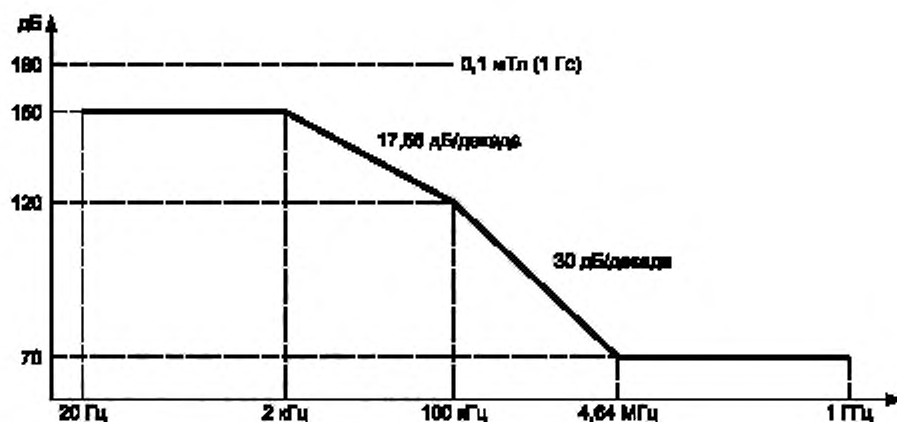
Рисунок В.50 — Минимальные уровни восприимчивости к помехам ближнего поля для модулей типов С и D (дБ относительно 1 нТл)
