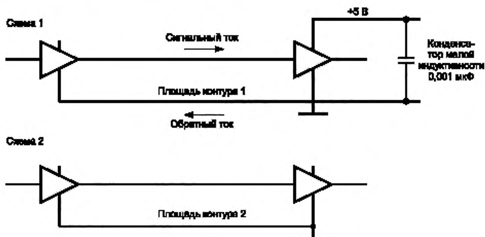
Рисунок П.1 — Типичные логические схемы
