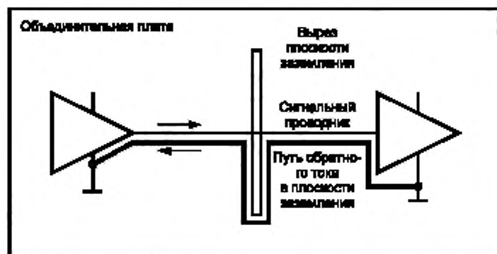
Рисунок П.2 — Площадь контура при наличии выреза в плоскости заземления
