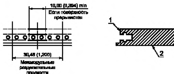
1 — опорная поверхность эжектора, должна быть токопроводящей; 2 — передний горизонтальный элемент
