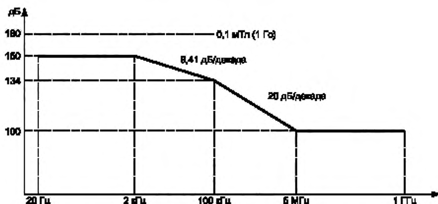
Рисунок В.49 — Минимальные уровни восприимчивости к помехам ближнего поля для модулей типов А и В (дБ относительно 1 нТл)
