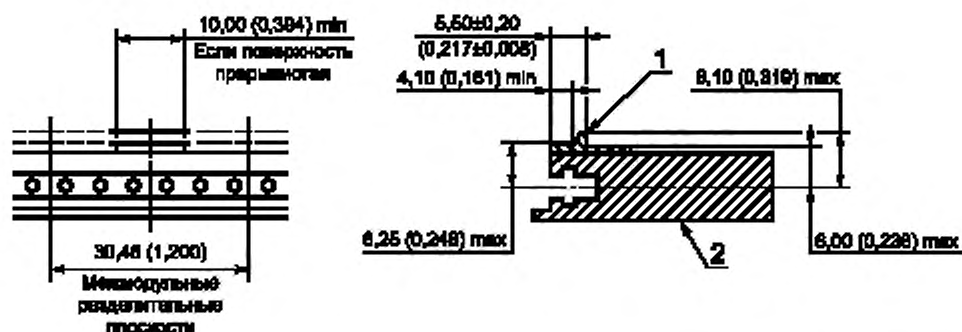
1 — опорная поверхность устройства установки; 2 — передний горизонтальный элемент
