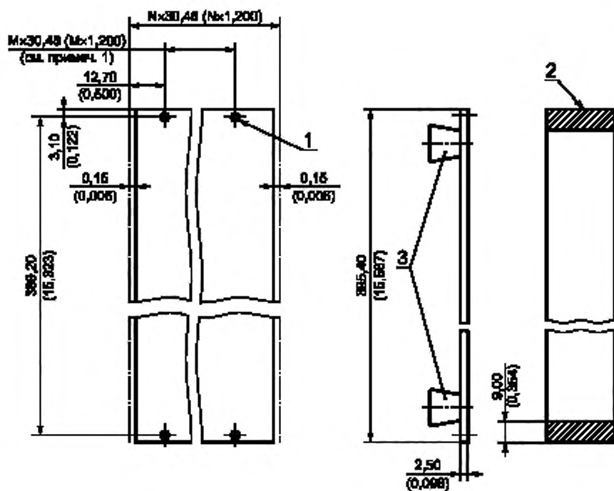
1 — см. рисунок В.23; 2 — минимальная зона корпусного электроконтакта; 3 — см. примечание 2
