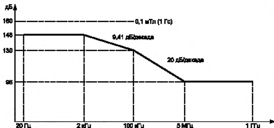
Рисунок В.47 — Максимальные уровни помех ближнего поля для модулей типов размеров А и В (дБ относительно 1 нТл)
