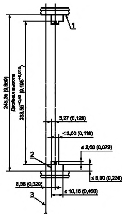
1 — горизонтальный элемент; 2 — направляющая; 3 — межмодульная разделительная плоскость
