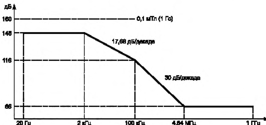
Рисунок В.48 — Максимальные уровни помех ближнего поля для модулей типов размеров С и D (дБ относительно 1 нТл)
