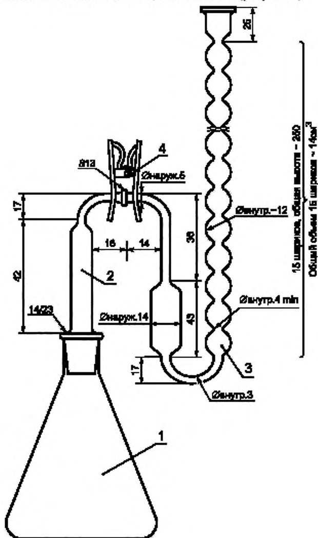
1 — реакционный сосуд; 2 — соединительная трубка; 3 — абсорбиционный сосуд; 4 — предохранительные зажимы
