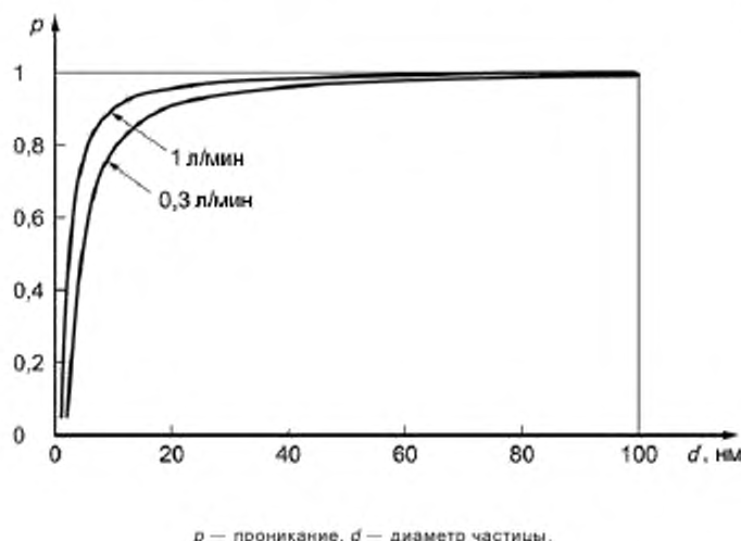
Рисунок 3 — Диффузионные потери, вычисленные для трубки длиной 1 м для двух значений расхода
