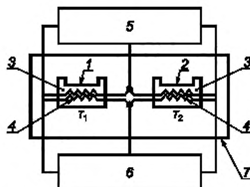
1 — положение испытуемого образца; 2 — положение эталонного тигля или эталонного образца; 3 — термометры; 4 — индивидуальные нагреватели; 5 — измерительный контур для T_{\text{specimen}} и T_{\text{ref}} ; 6 — устройство для компенсации мощности; 7 — теплоотводящее устройство; T_1 — температура вблизи образца ( T_{\text{specimen}} ); T_2 — температура вблизи эталонного тигля или эталонного образца ( T_{\text{ref}} )
