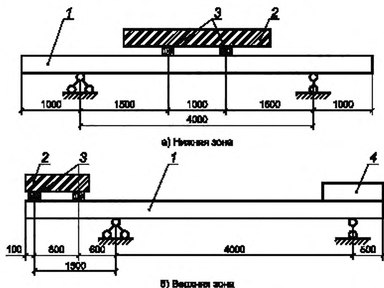
1 — испытательная плита; 2 — контрольная нагрузка; 3 — деревянные брусья сечением 10 × 10 см; 4 — пригрузочный балласт P \approx 2,0 тс
