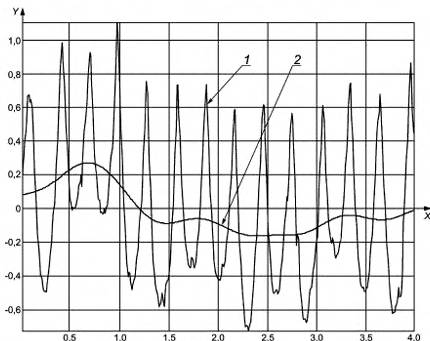
1 — профиль до фильтрации; 2 — профиль после фильтрации; X — длина, мм; Y — высота, мкм
