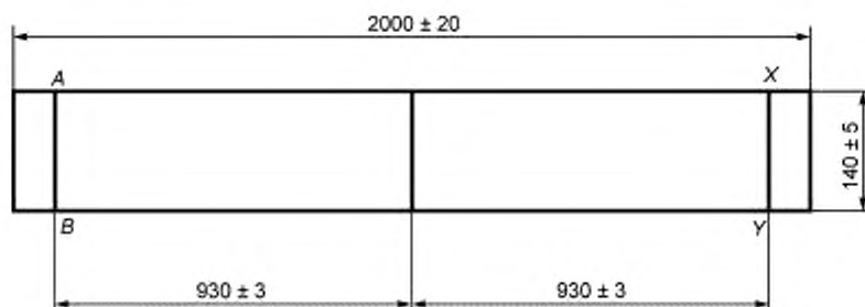
Рисунок 2 — Диаграмма для прочерчивания линий на ремне
