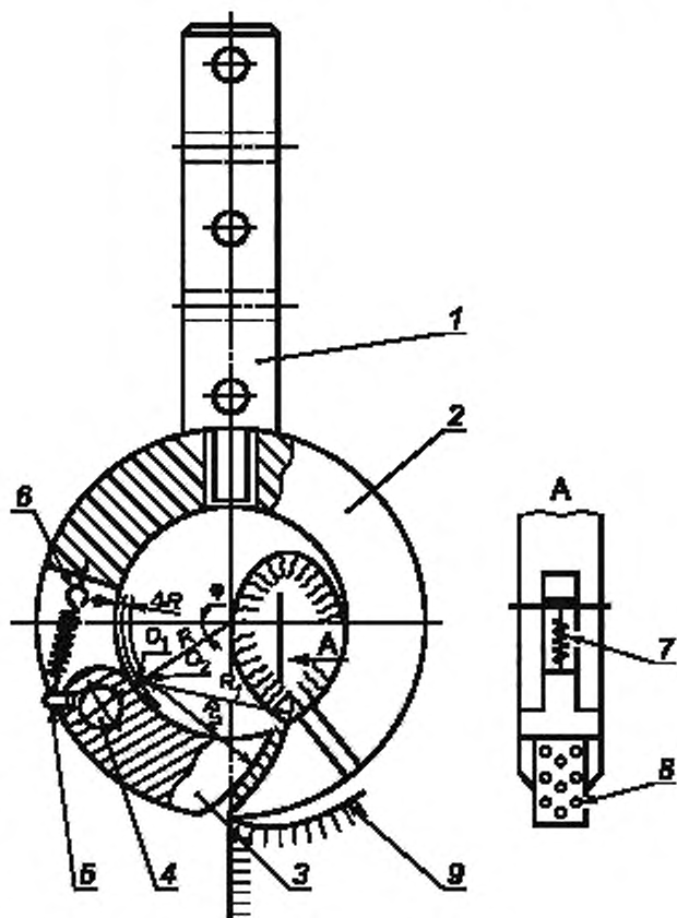
1 — хвостовик, 2 — кольцо; 3 — губка подвижная, 4 — ось, 5 — шпилька; 6 — штифт; 7 — пружина; 8 — игла; 9 — шкала или изделие
