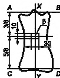
Рисунок 7 — Разметка шкурок шириной до 16 см
