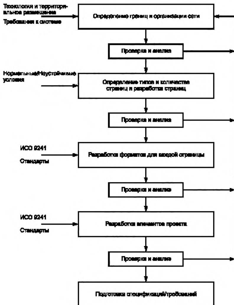
Рисунок А.1 — Процесс структурирования информации
