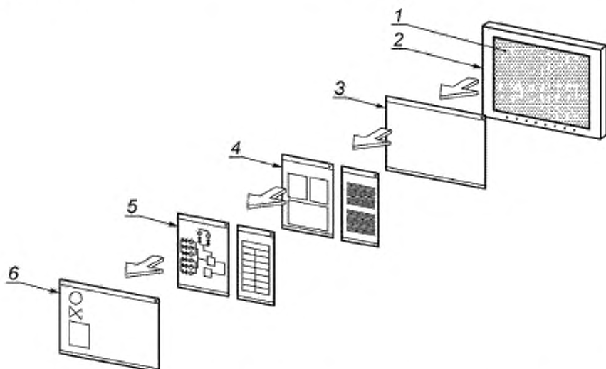
1 — экран дисплея; 2 — дисплей; 3 — страница (все представлено на единственном экране дисплея); 4 — окно (одно окно может занимать весь экран дисплея); 5 — формат (например, мнемосхема, гистограмма, кривая тренда); 6 — элемент (например, ярлык, метка)
