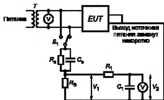
Рисунок 5 — Испытательная установка
