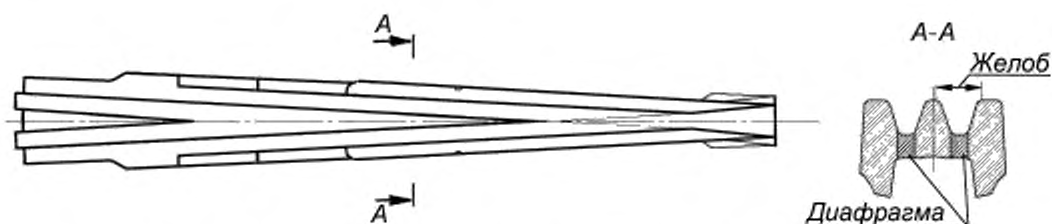
Рисунок 3.3 — Литой сердечник сборной крестовины и его поперечное сечение в зоне перекачивания
