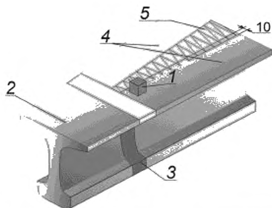
Рисунок В.3 — УЗК продольного сварного шва сварки рельсовых окончаний в области подошвы
