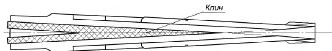
Рисунок 3.6 — Клин литого сердечника сборной крестовины
