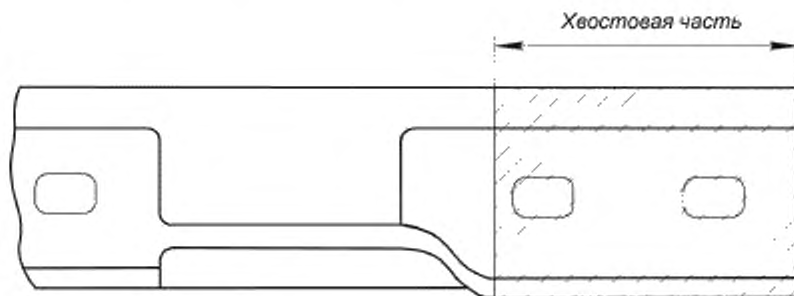
Рисунок 3.13 — Хвостовая часть литого сердечника сборной крестовины
