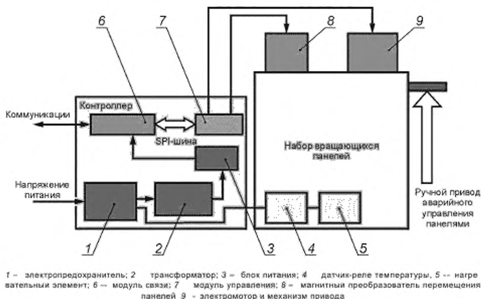
Рисунок А.2 — Функциональная схема электромеханического дорожного знака переменной информации
