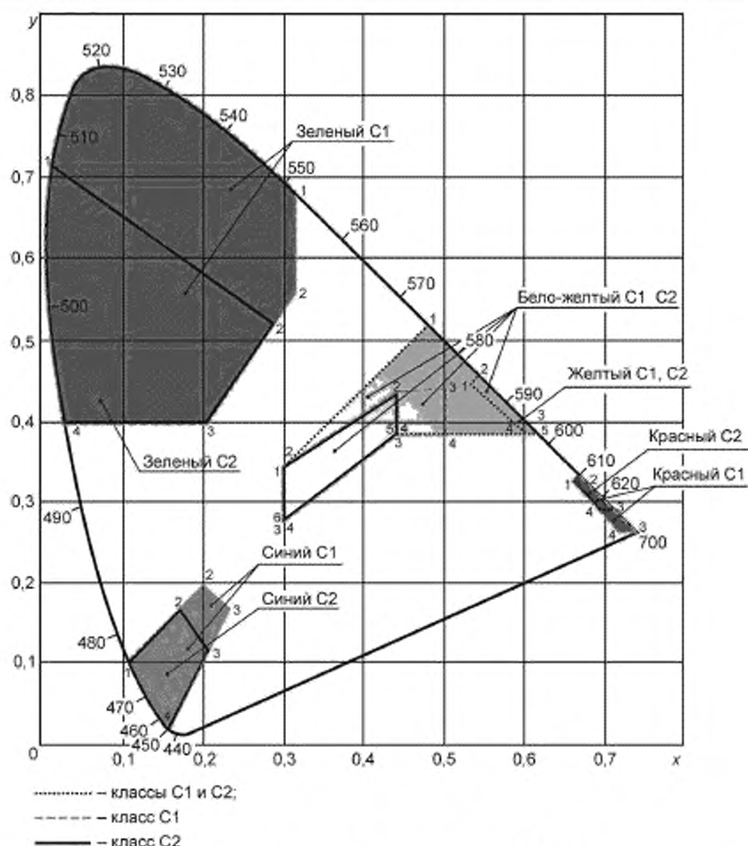
Рисунок 1 — Допустимые области цветности для цветов классов C1 и C2 на диаграмме цветности
