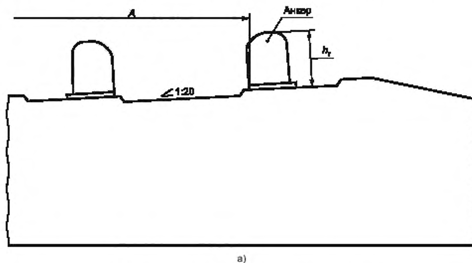
Рисунок 7, лист 1 — Подрельсовая часть шпал типа II
