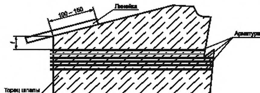
Рисунок 21 — Схема определения толщины t защитного слоя бетона
