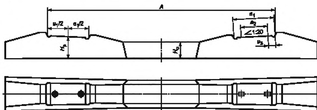
Рисунок 3 — Спальи типа III
