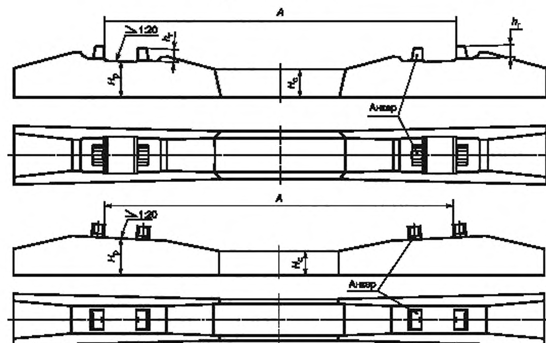
Рисунок 2 — Схема шпал типа II
