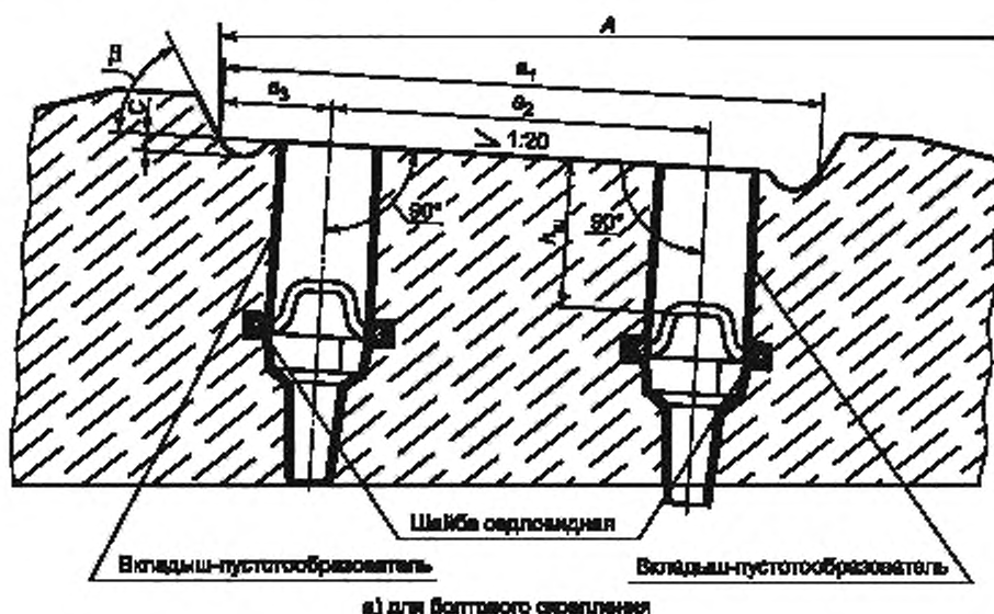
Рисунок 6, лист 1 — Подрельсовая часть шпал типа III
