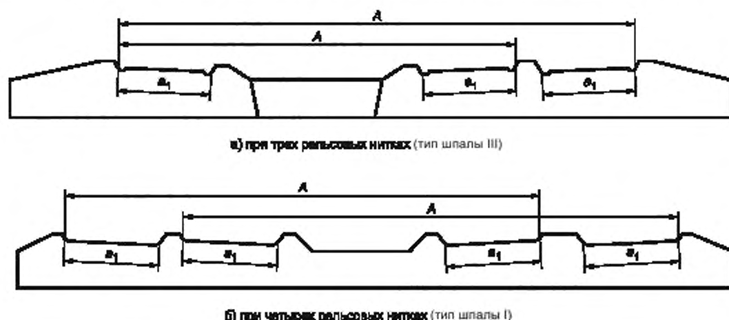
Рисунок 4 — Спальи с совмещенной колеёй разной ширины
