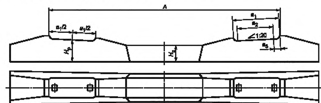
Рисунок 1 — Схема шпал типа I
