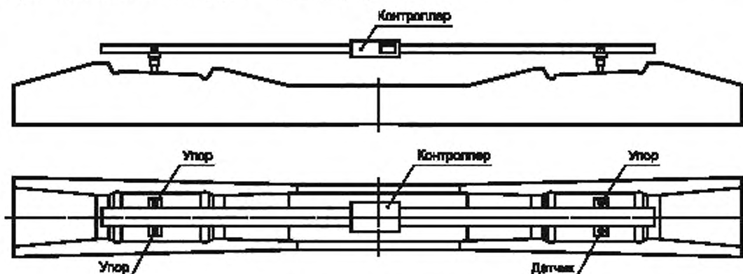
Рисунок 19 — Схема контроля пропеллерности подрельсовых площадок прибором ПКП-01Ш
