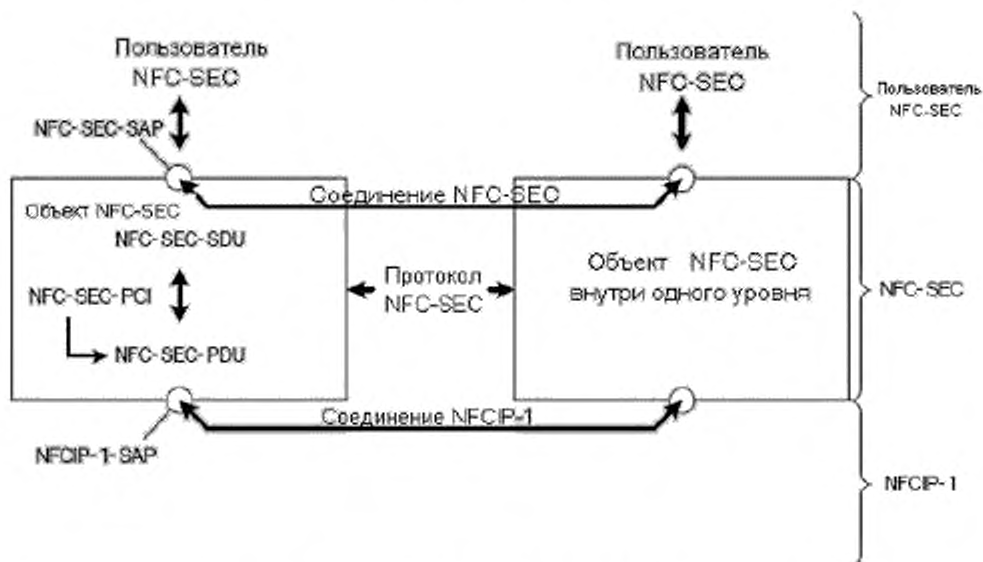
Рисунок 1 – Архитектура NFC-SEC
