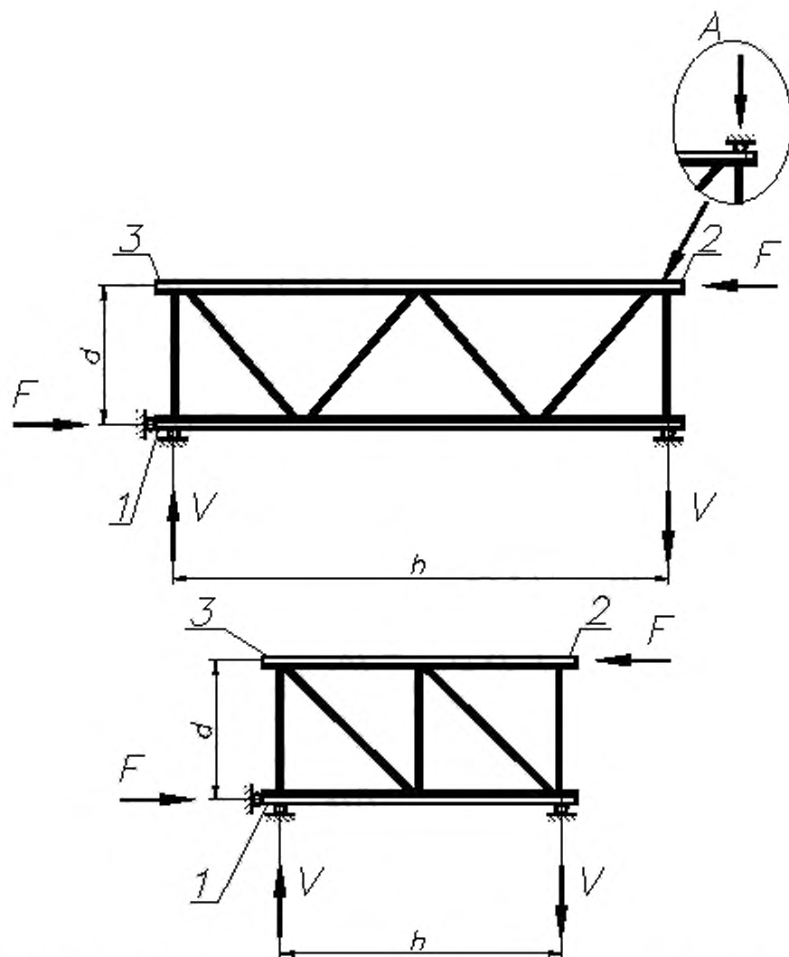
Рисунок A.13 — Порядок проведения испытаний для оценки жесткости рамы при действии поперечной силы
