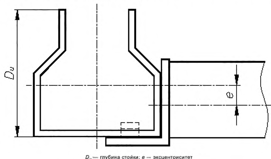
Рисунок 11 — Эксцентриситет в Y-направлении
