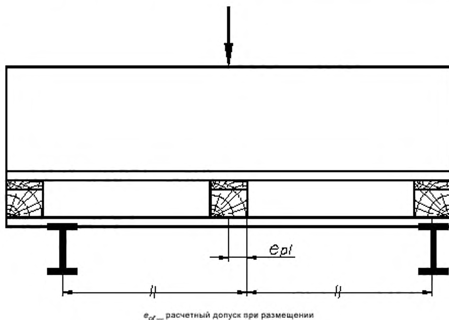
Рисунок Е.1 — Эксцентриситет нагрузки
