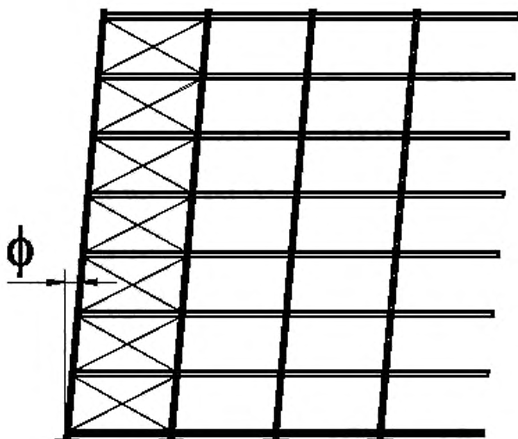
Рисунок 8 — Общие отклонения от вертикальной плоскости
