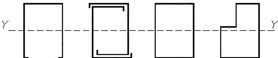
Рисунок 19 — Примеры балок, для которых маловероятна потеря устойчивости плоской формы изгиба при небольшом соотношении высоты к ширине и в зависимости от длины балки
