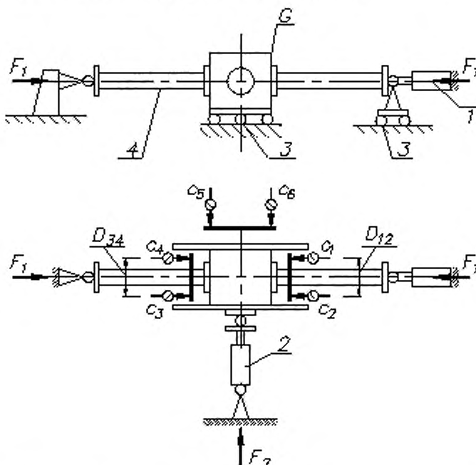
1 и 2 — нагружающие устройства; 3 — роликовый подшипник; 4 — образец стойки; C_1 - C_6 — датчики; D_{12} и D_{34} — расстояния между измерительными приборами; F_1 и F_2 — прикладываемые силы; G — бетонный блок
