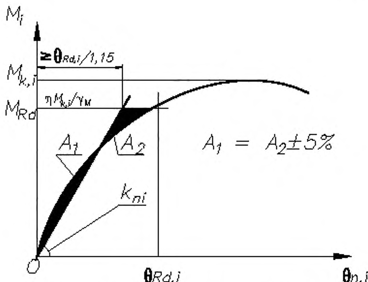
Рисунок А.6 — Обработка значений жесткости кронштейна балки
