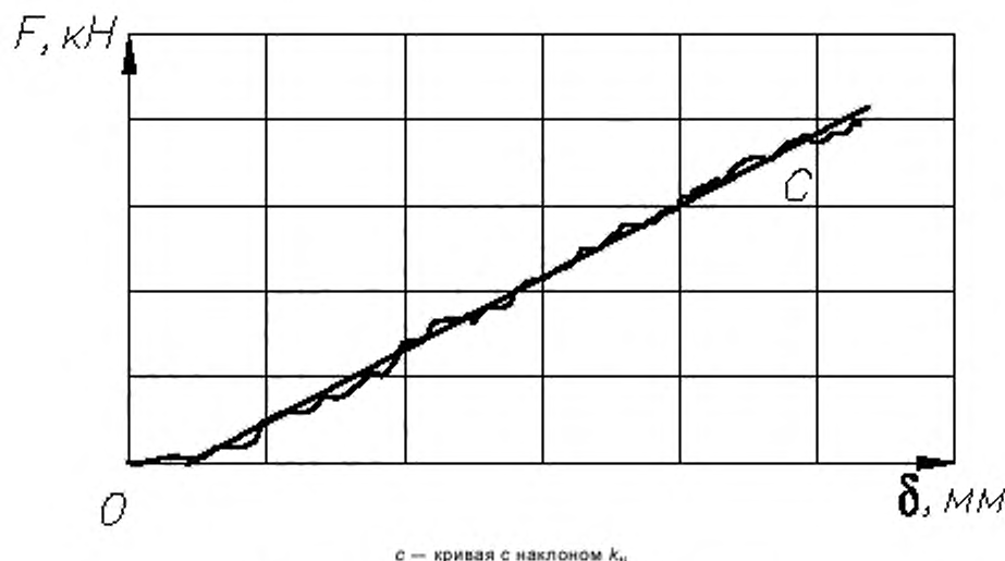
Рисунок А.14 — Кривая нагружения – деформации
