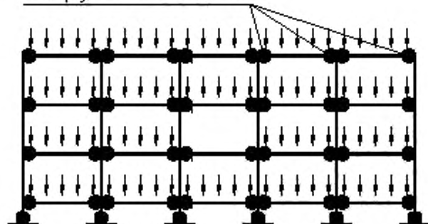
Рисунок 27 — Схемы нагружения для расчета в X-направлении
