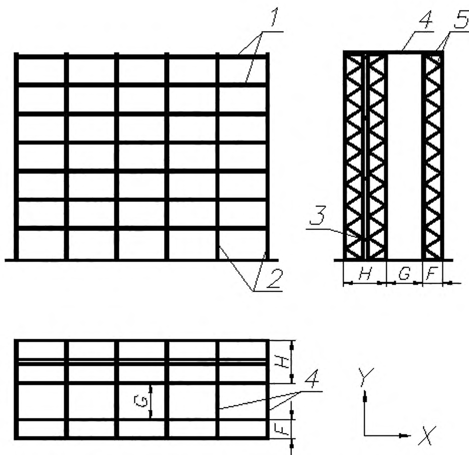
1 — балки; 2 — рамы; 3 — межрамные связи; 4 — связь над рабочим коридором (при необходимости); 5 — раскосная система рамы; F — ширина одиночного ряда; G — ширина рабочего коридора; H — ширина двойного ряда
