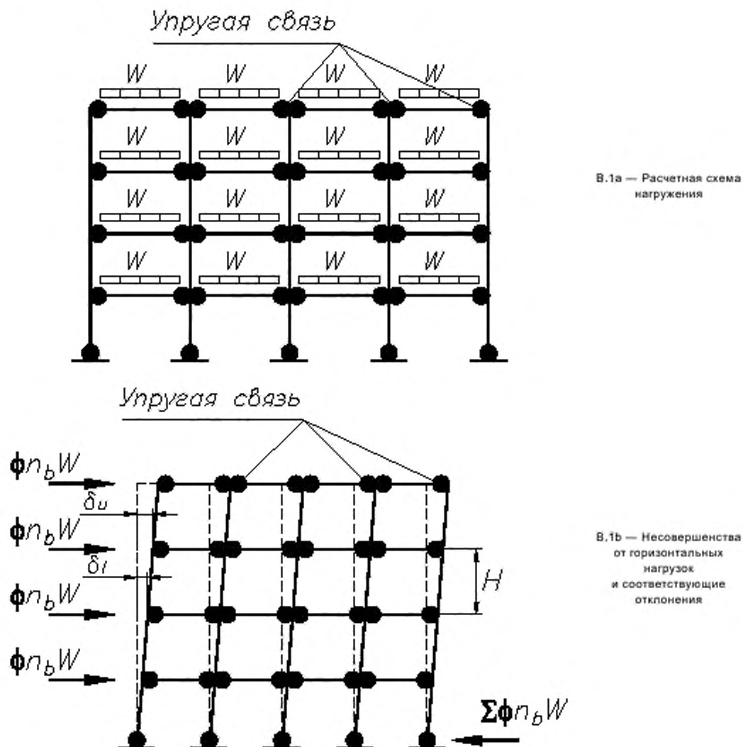
Рисунок В.1 — Схема метода увеличенных моментов
