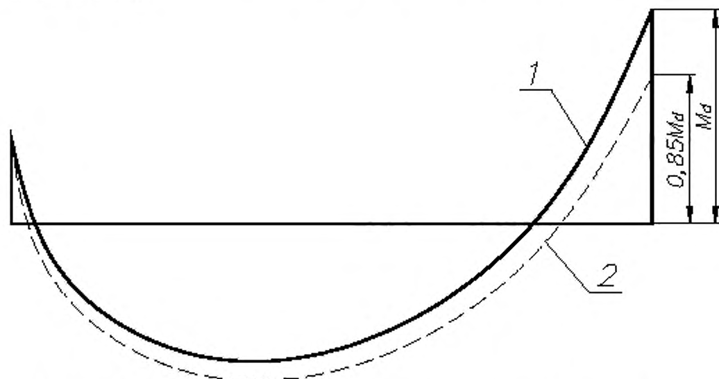
Рисунок 17 — Перераспределение моментов балок
