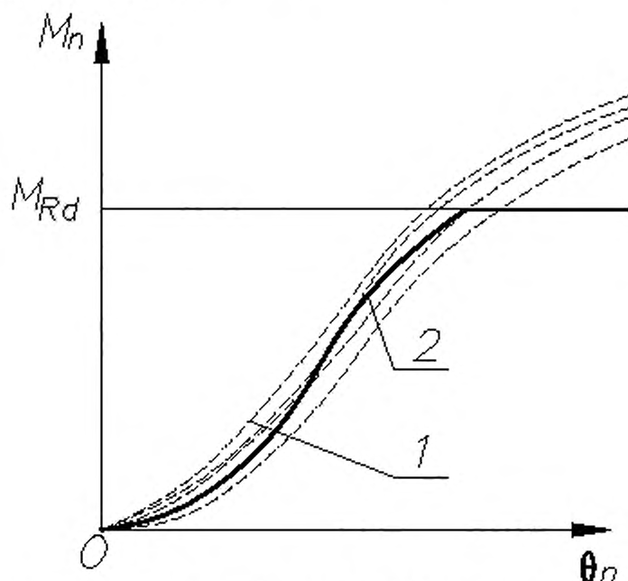
Рисунок А.7 — Определение «средней» кривой зависимости момент-поворот
