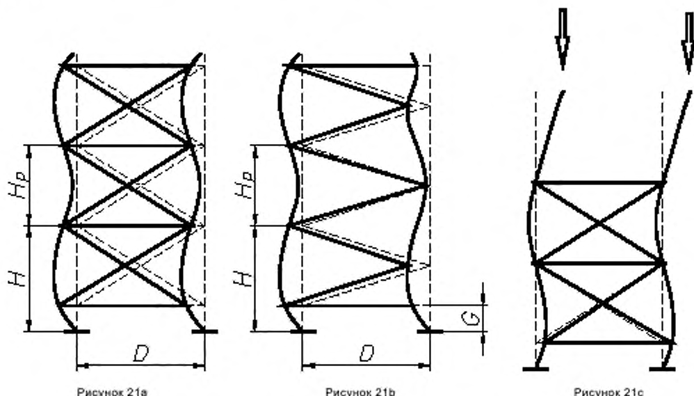
D — расстояние между стойками в раме; G — эксцентриситет; H — высота уровня; H_p — наибольшая длина стержня между узлами крепления раскосов
