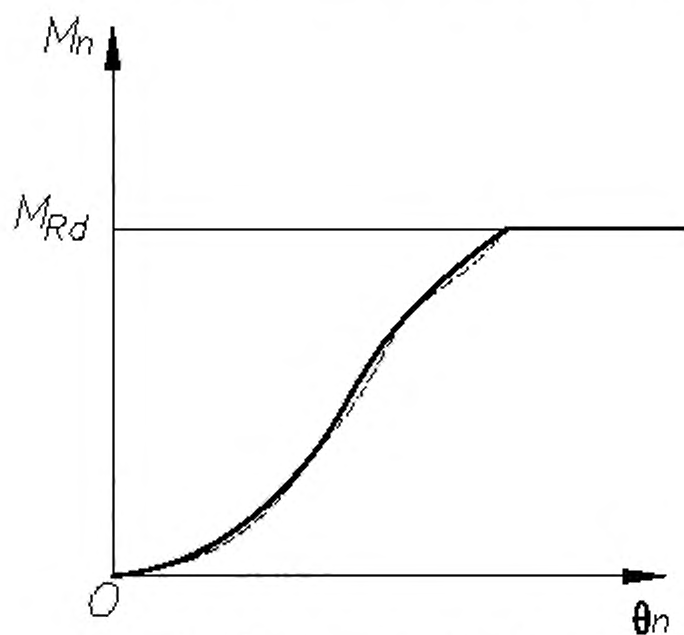
Рисунок А.8 — Типовая линейаризация средней кривой
