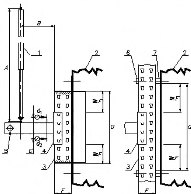
1 — шток гидроцилиндра испытательной установки; 2 — рама испытательной установки; 3 — элемент стойки; 4 — кронштейн балки; 5 — ограничение поворота балки в боковом направлении; 6 — зажим; 7 — прокладка для зазора; A \geq 750 мм; B = 400 мм; C — расстояние между датчиками перемещения; d — измерительные приборы; F — ширина плоскости стойки; G — длина испытываемого образца;
