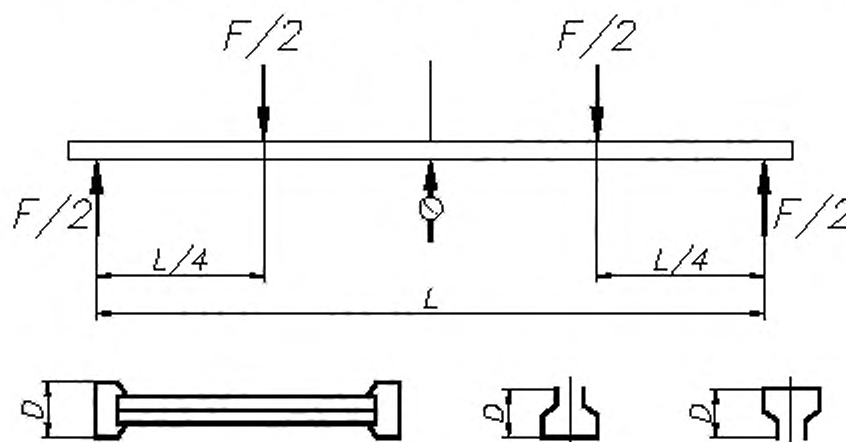
Рисунок А.15 — Порядок проведения испытаний
