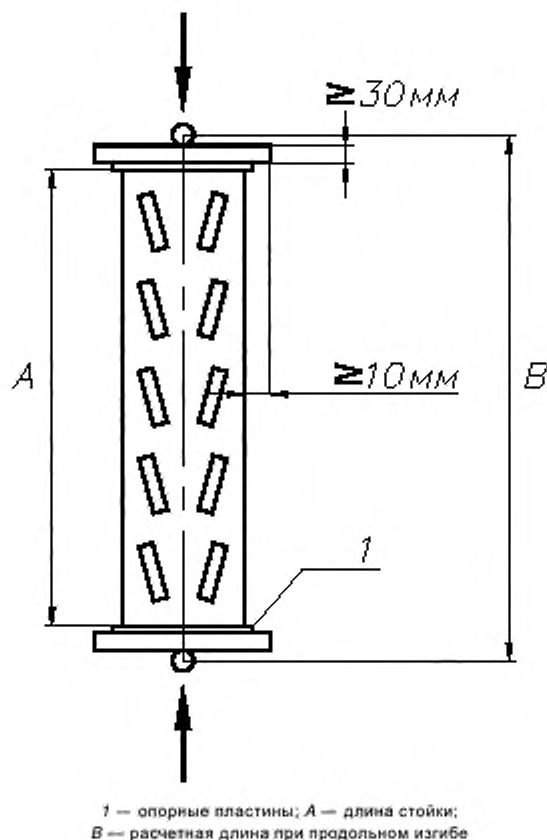
Рисунок А.2 — Порядок проведения испытаний короткой стойки на сжатие
