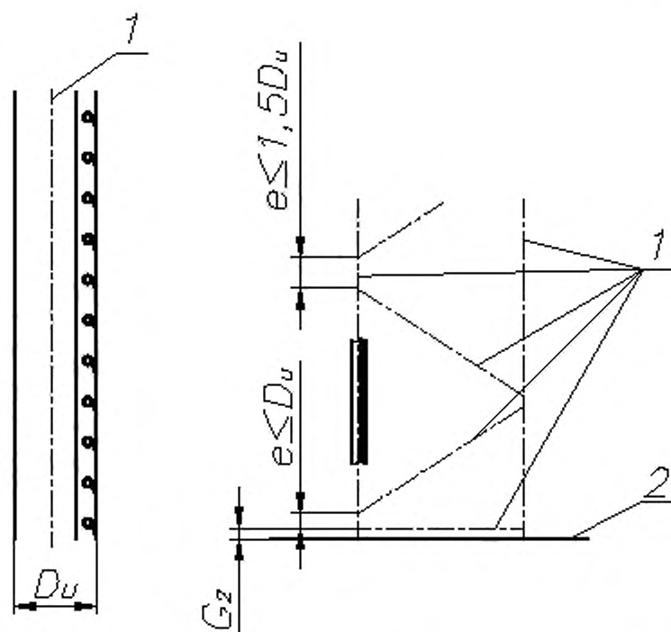
Рисунок 10b — Эксцентриситеты раскосной системы рамы
