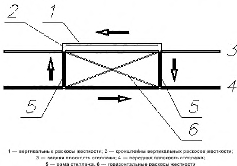
Рисунок 6 — Направления усилий от действия крестовых раскосов жесткости в одиночном ряду стеллажей
