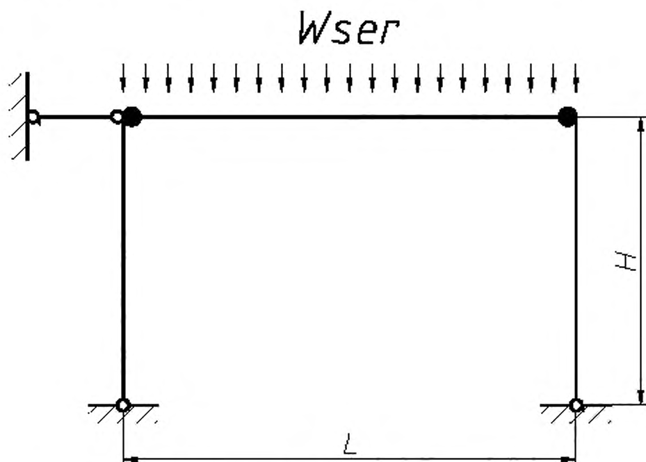
Рисунок 18 — Схема для предварительного расчета прогиба балки
