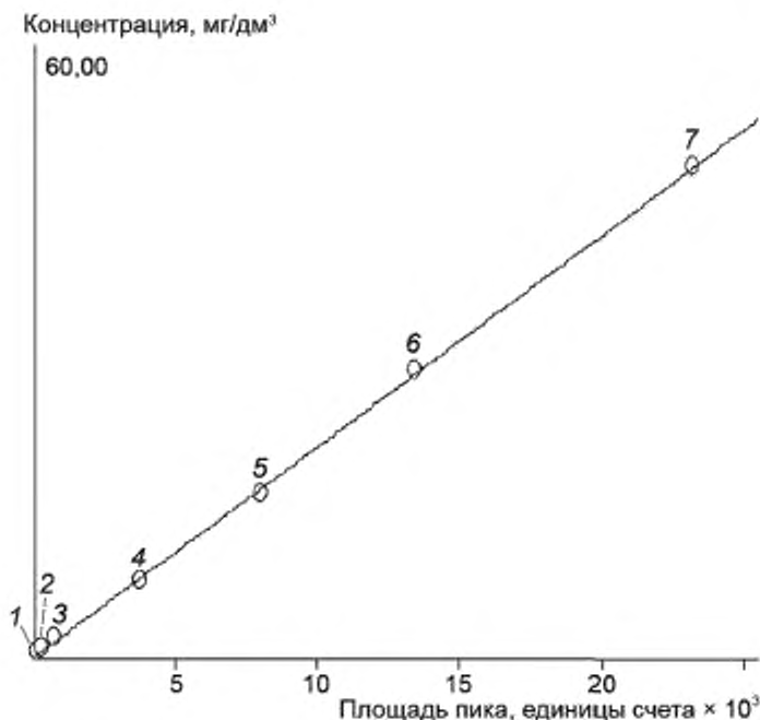
Рисунок 3 — Типичный калибровочный график сульфата
