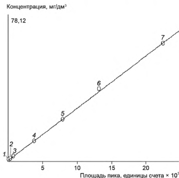
Рисунок 2 — Типичный калибровочный график хлорида
