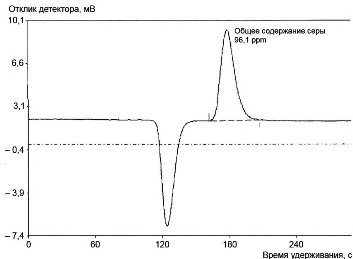
Рисунок 1 — Типовая хроматограмма
