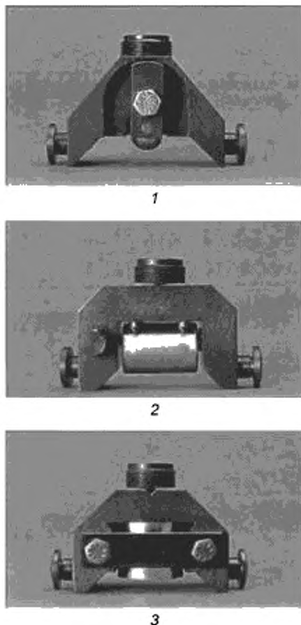
1 — точечный контакт, 2 — линейный контакт, 3 — плоскостной контакт
