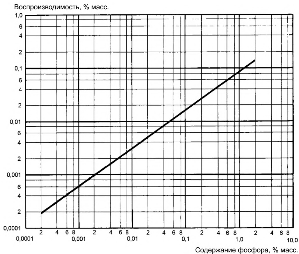
Рисунок 3 — Воспроизводимость результатов испытаний, полученных фотометрическим методом
