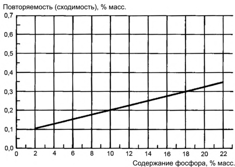
Рисунок 2 — Повторяемость (сходимость) результатов испытаний, полученных гравиметрическим методом
