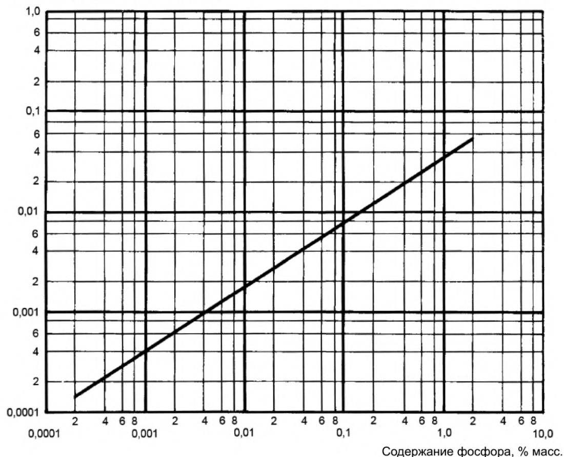
Рисунок 1 — Повторяемость (сходимость) результатов испытаний, полученных фотометрическим методом
