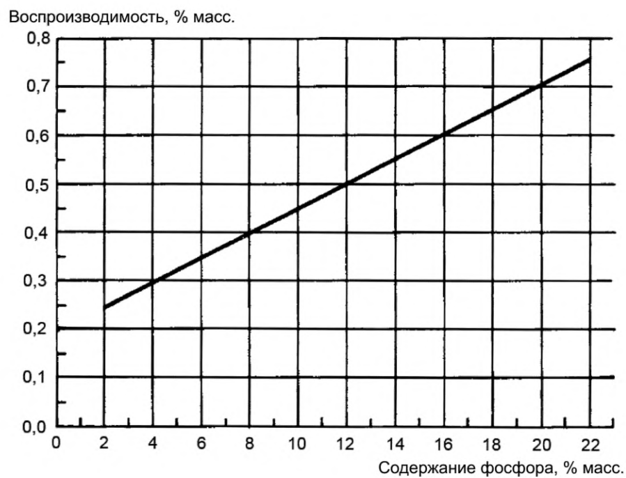
Рисунок 4 — Воспроизводимость результатов испытаний, полученных гравиметрическим методом
