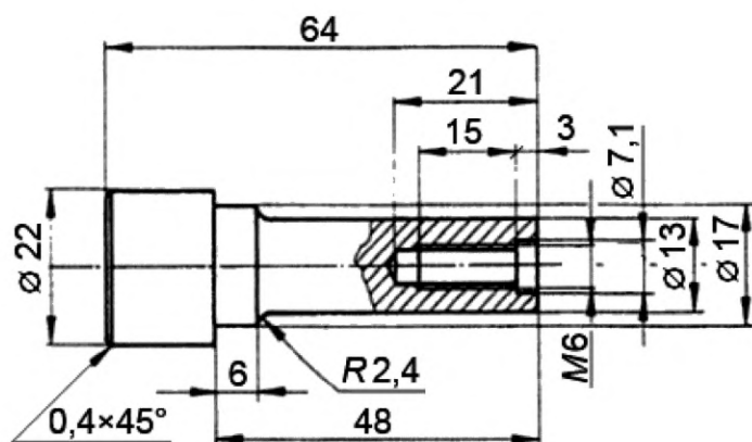
Держатель стержня, тип 2
