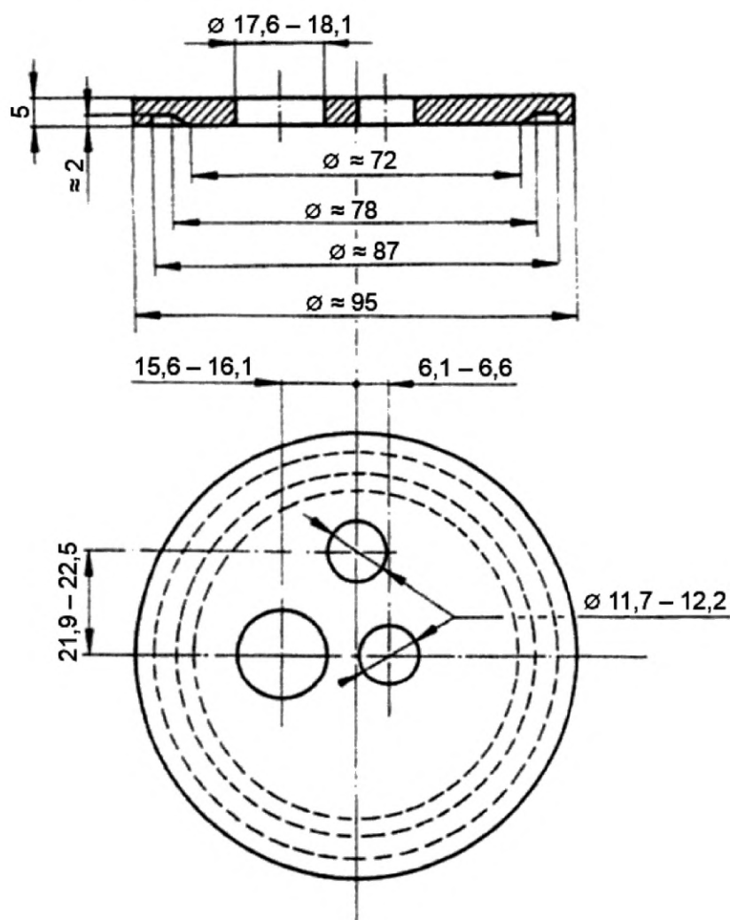
Рисунок 2 — Крышка стакана
