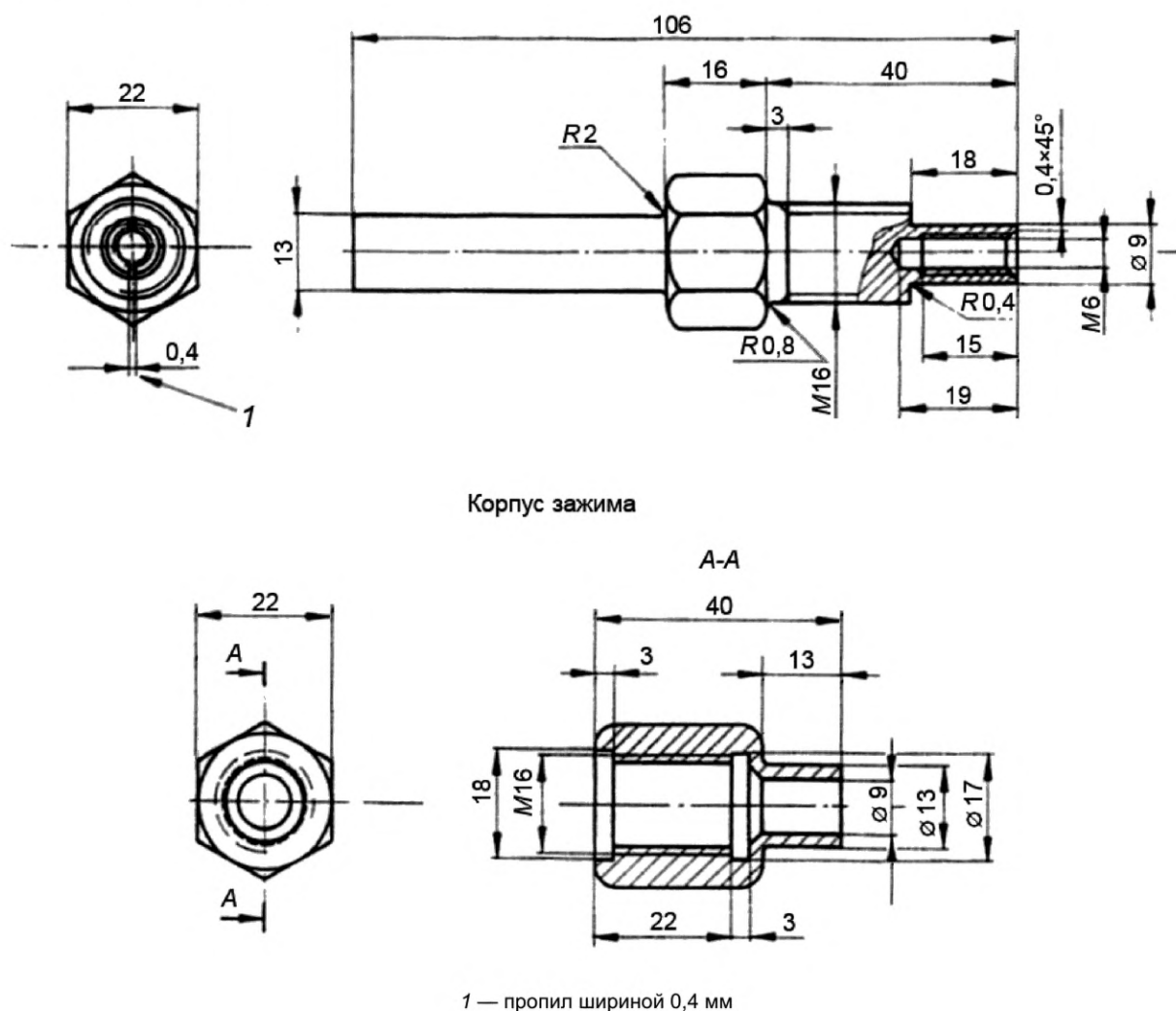
Рисунок 4 — Зажим для шлифовки стержней для испытания
