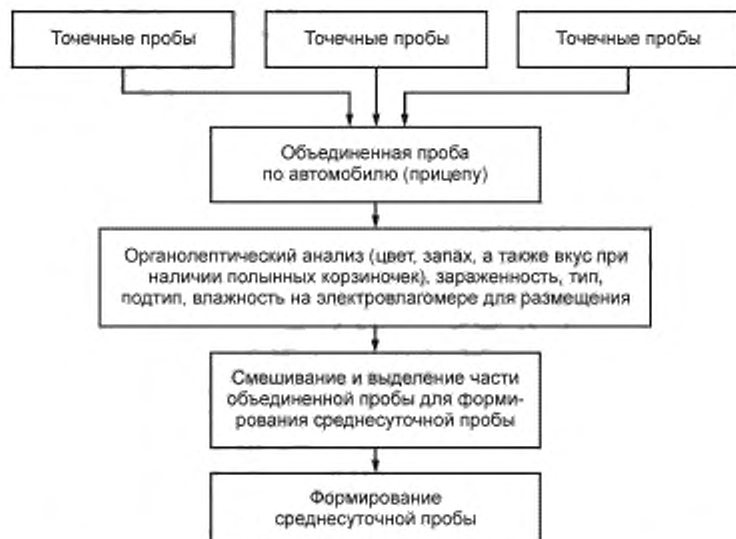
Рисунок 1 — Схема формирования среднесуточной пробы при доставке зерна автомобильным транспортом
