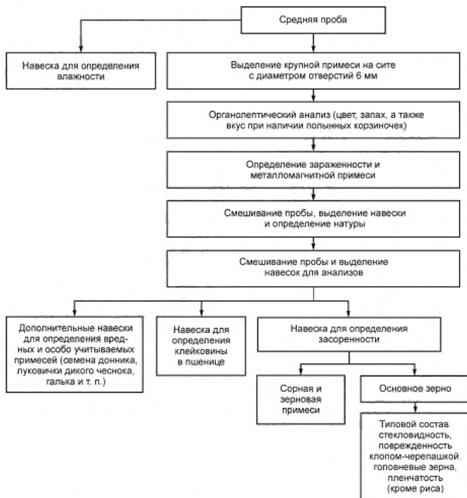
Рисунок 2 — Схема проведения лабораторного анализа средней пробы
