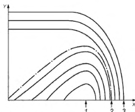
X — P_1 , выражается в килопаскалях (фунтах на квадратный дюйм); Y — q_g , выражается в СКМС (СКФС); 1 — P_{vOT} ; 2 — P_{vOT} ; 3 — P_{vST}
