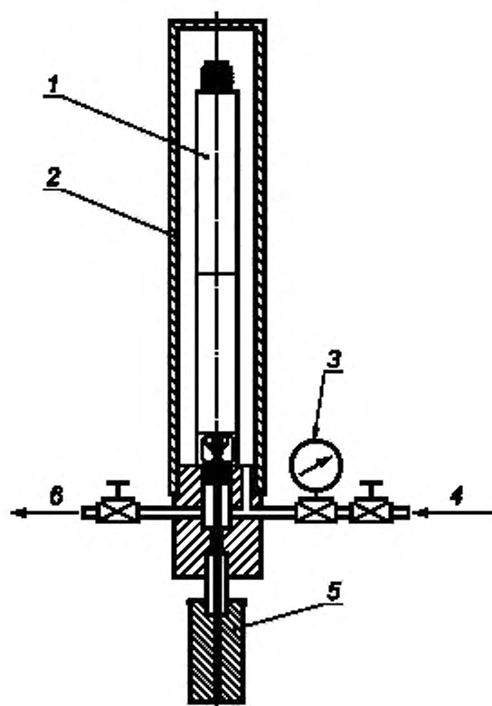
1 — устройство для регулирования дебита; 2 — испытательная установка; 3 — манометр; 4 — прибор для контроля газа; 5 — ЛДПС; 6 — выпуск газа
