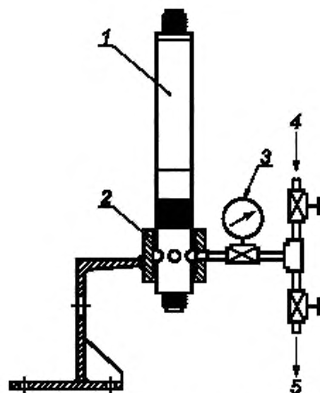
1 — устройство для регулирования дебита; 2 — кольцевое приспособление, 3 — манометр; 4 — подводящий трубопровод, 5 — сравнение давления
