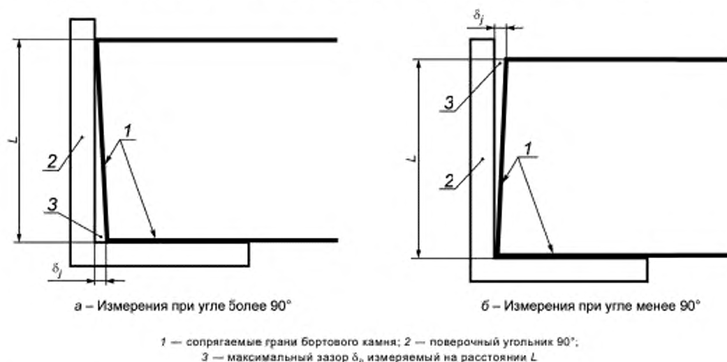
Рисунок 1 — Схема контроля взаимной перпендикулярности граней бортового камня
