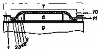
Рисунок 3 – Схема формования пластин в автоклаве
