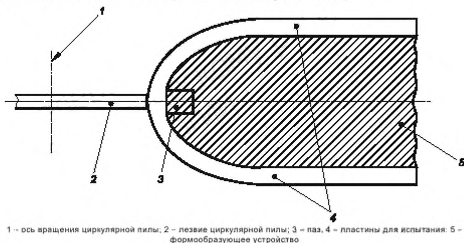
Рисунок 4 – Извлечение пластин для испытания из формообразующего устройства
