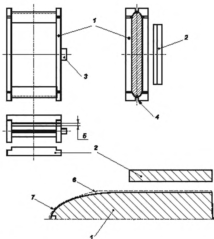
1 – плита; 2 – внешние части; 3 – шпindelный узел; 4 – паз; 5 – толщина намотки, 6 – силиконовый или резиновый уплотнитель; 7 – ролинг
