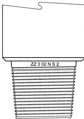
Рисунок 5 — Маркировка идентификации на основании штифта
