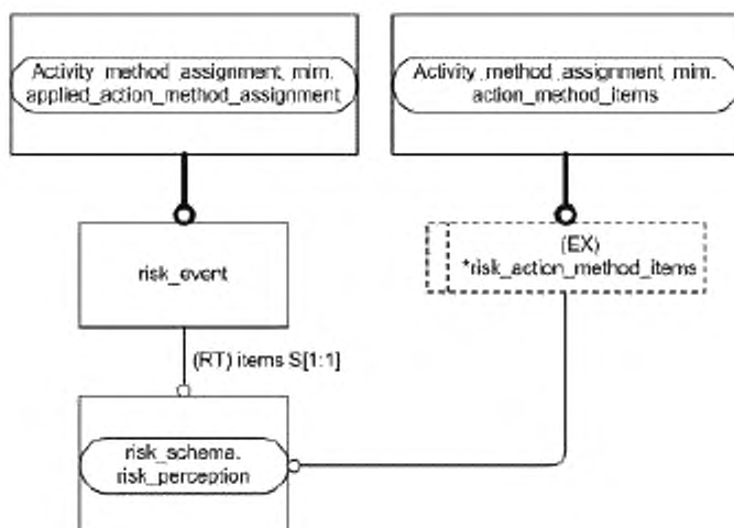
Рисунок D.2 – Представление IMM на уровне объектов в формате EXPRESS-G (диаграмма 1 из 1)
