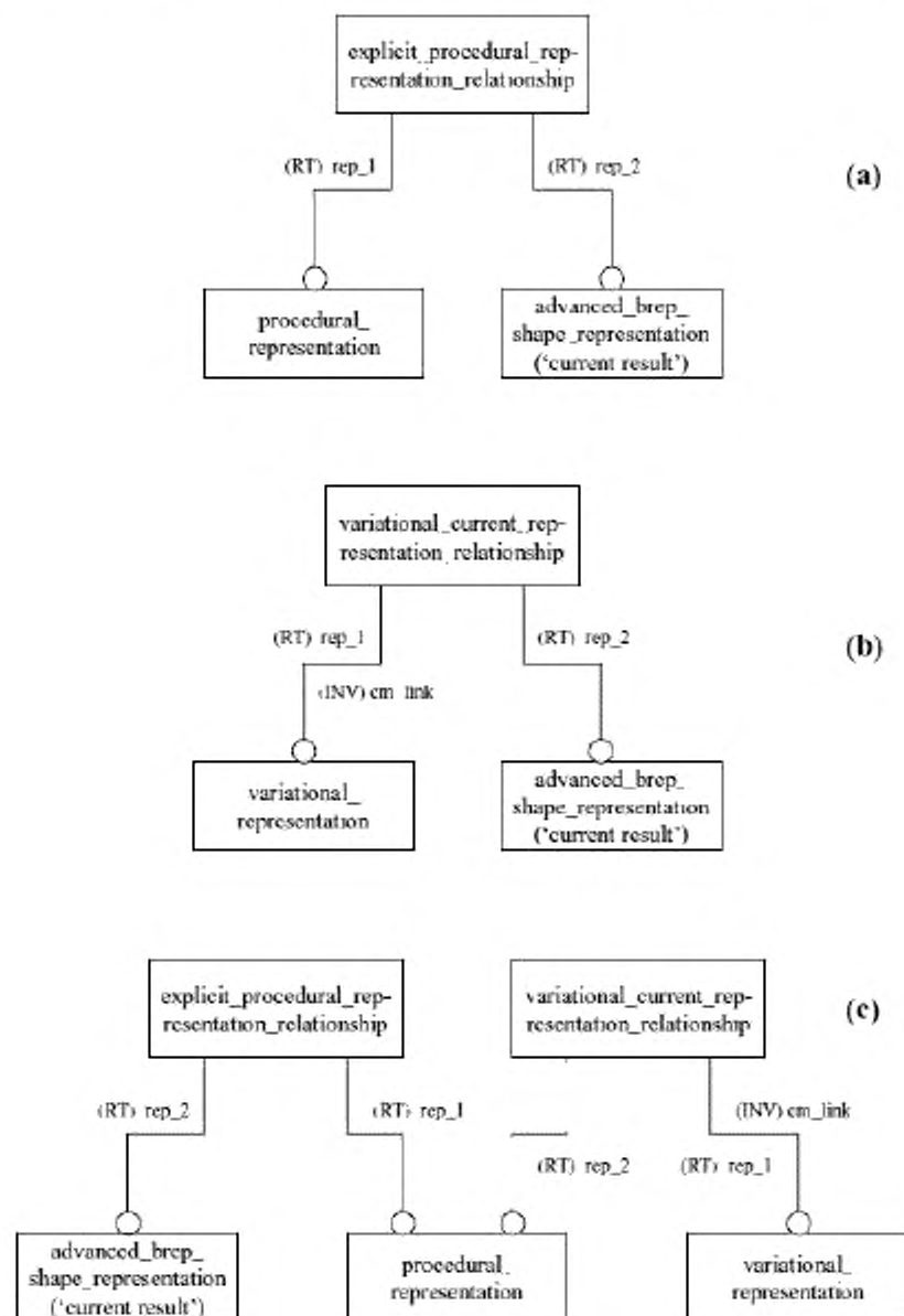
Рисунок Е.1 – Взаимосвязи между экземплярами процедурной, вариационной и явно заданной моделей для комбинаций (a) – без вариационной модели, (b) – без процедурной модели и (c) – наличие всех трех моделей
