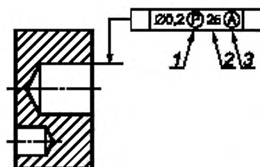
1 — указание на то, что допуск относится к выступающему элементу; 2 — длина выступающего нормируемого элемента; 3 — указание на то, что нормируемый элемент является средним элементом
