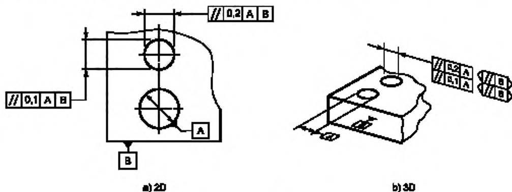
Рисунок 23 — Указание на чертеже
