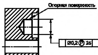
Рисунок 57 — Опорная поверхность выступающего элемента
