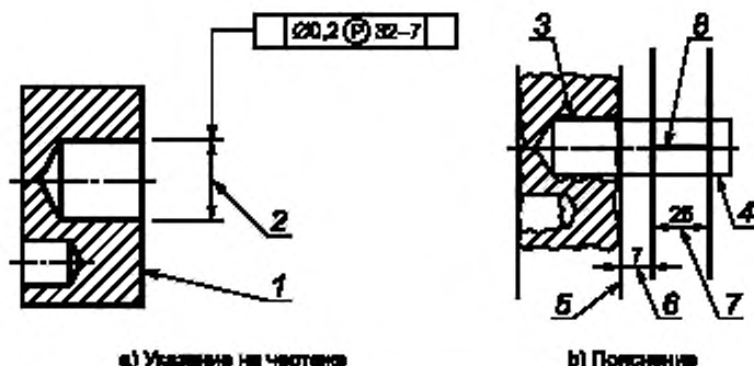
а) Указание на чертеже б) Пояснение 1 — опорная поверхность; 2 — указание на то, что нормируемым элементом является средний элемент (эквивалентно знаку \text{A} ); 3 — реальный элемент; 4 — продолженный элемент; 5 — опорная плоскость; 6 — смещение; 7 — длина нормируемого элемента; 8 — выступающий нормируемый элемент
