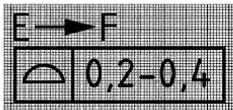
Рисунок С.6 — Знак «от ... до»
