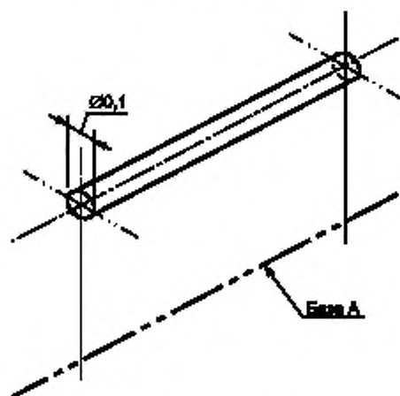
Рисунок 26 — Пояснение к рисунку 25
