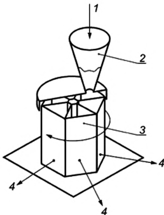
1 — подающий механизм; 2 — воронка; 3 — вращающийся приемник; 4 — разделитель проб
