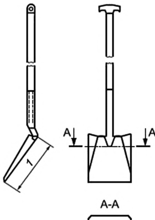
Рисунок 4 — Пример совка
