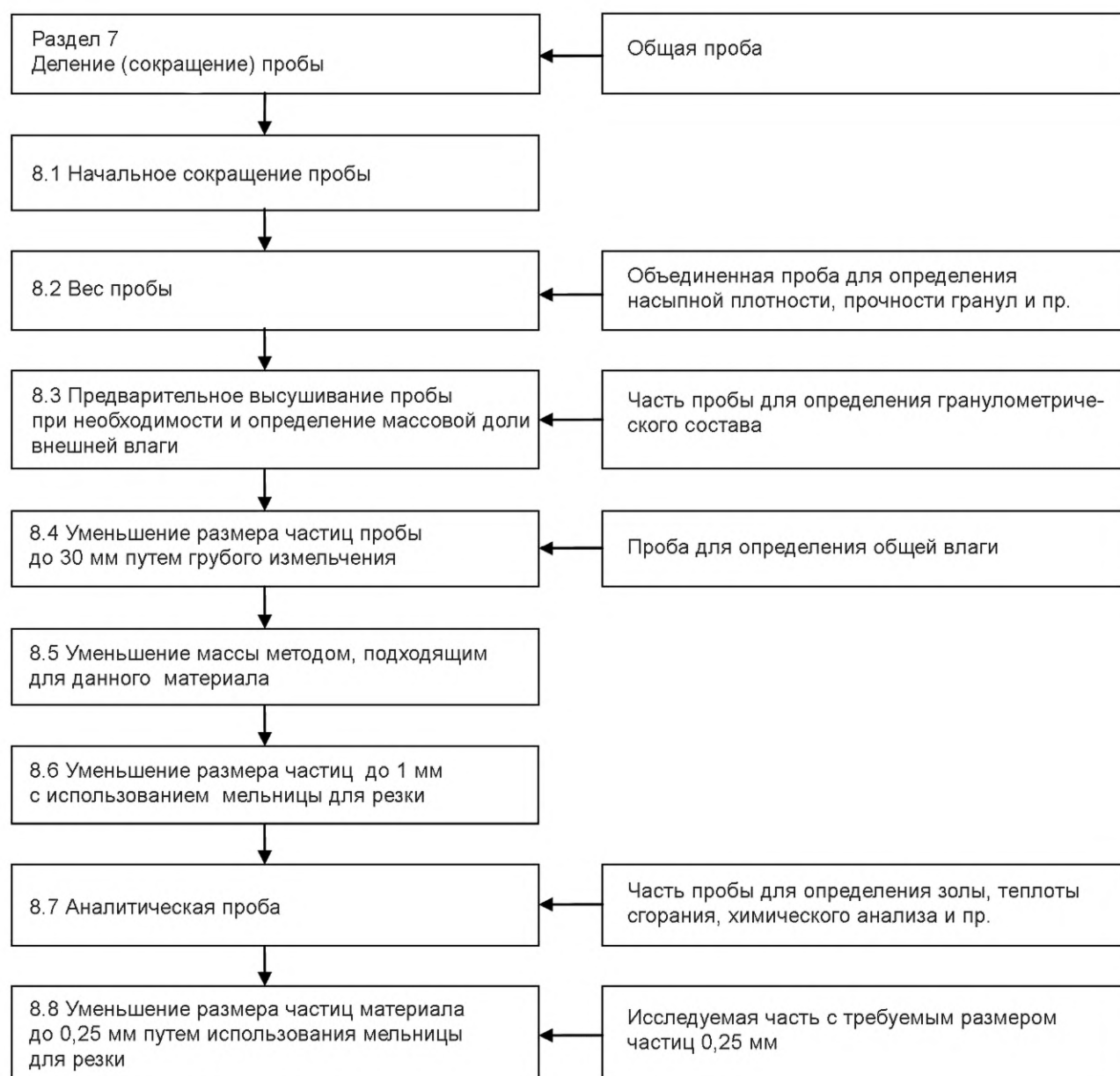
Рисунок 5 — Схема сокращения пробы
